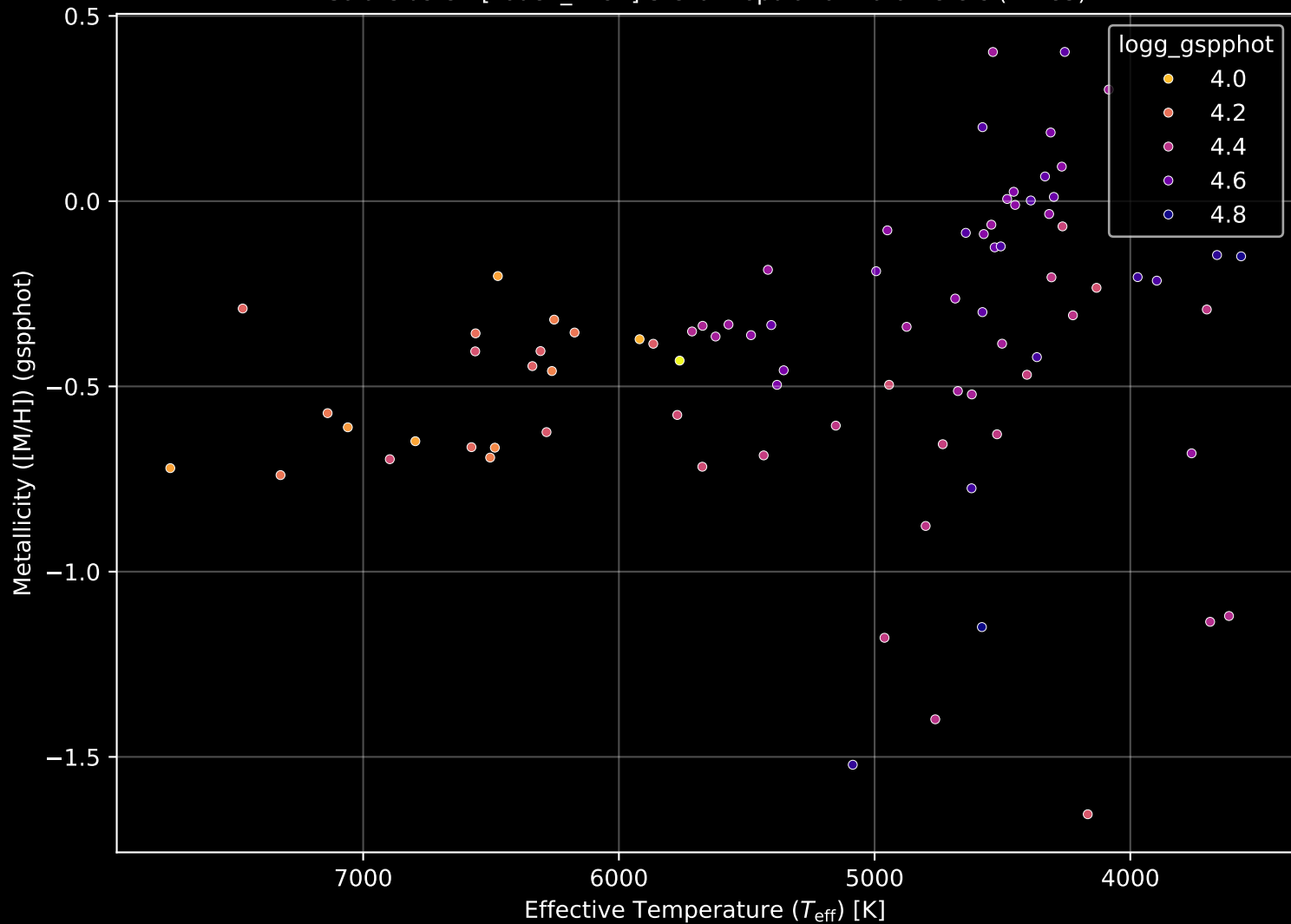
Gaia Cluster: [Loden_1194] Stellar Population Parameters (n= 85)
