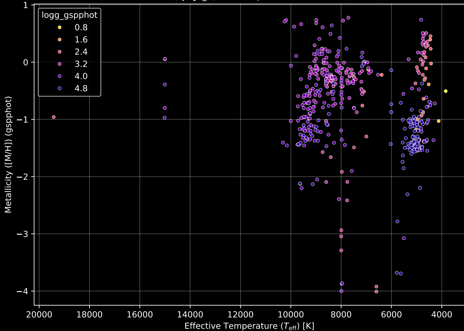
Gaia Cluster: [Lynga_9] Stellar Population Parameters (n= 497)
