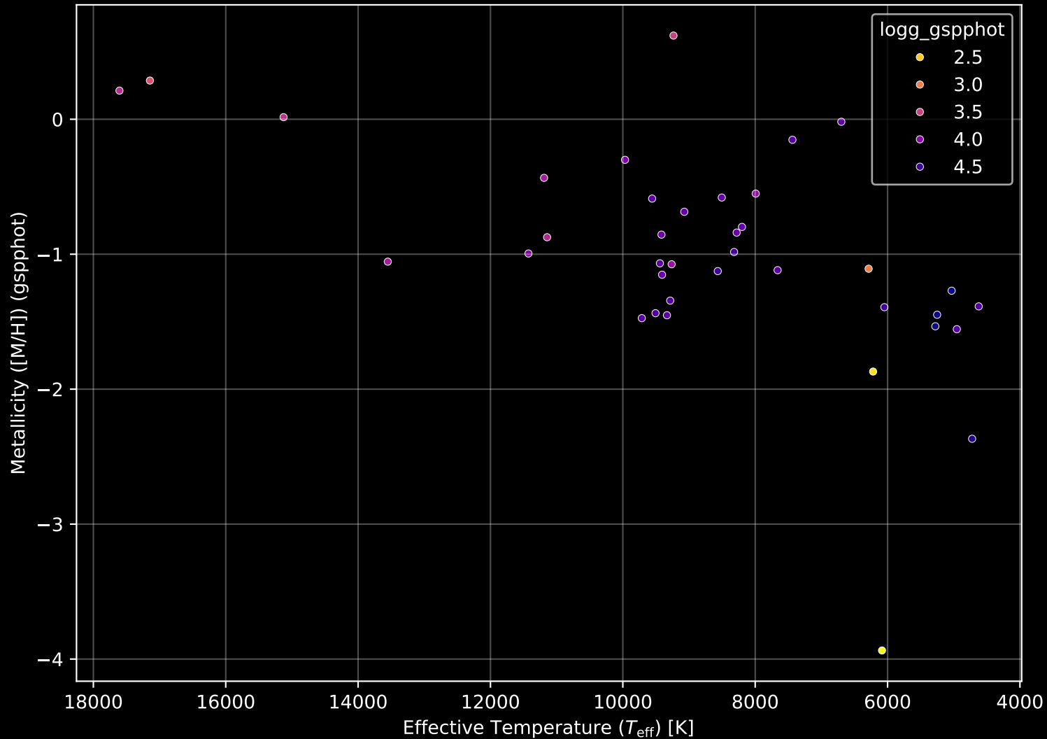
Gaia Cluster: [Markarian_50] Stellar Population Parameters (n= 38)
