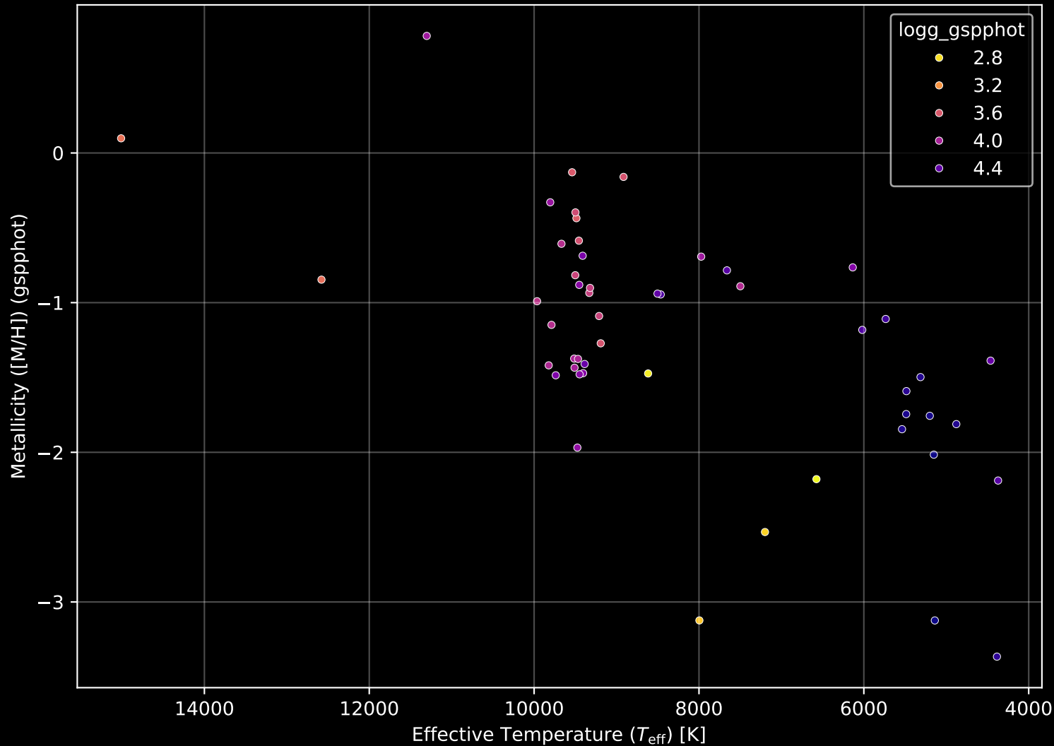
Gaia Cluster: [Mayer_3] Stellar Population Parameters (n= 51)
