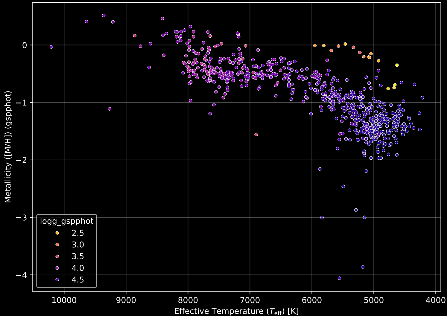
Gaia Cluster: [Melotte_71] Stellar Population Parameters (n= 639)
