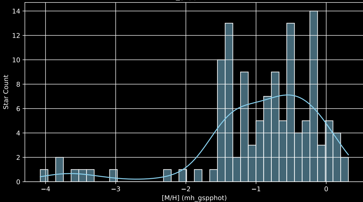
Gaia Cluster: [Muzzio_1 [M/H] (mh_gspphot) (n= 124)
