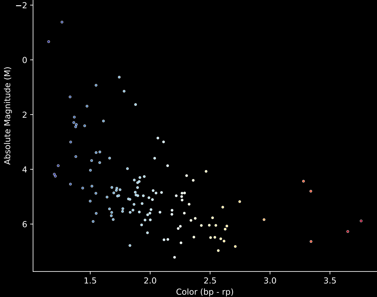
Gaia Cluster: [Muzzio_1] Stars (n= 124) Hertzsprung-Russel Diagram
