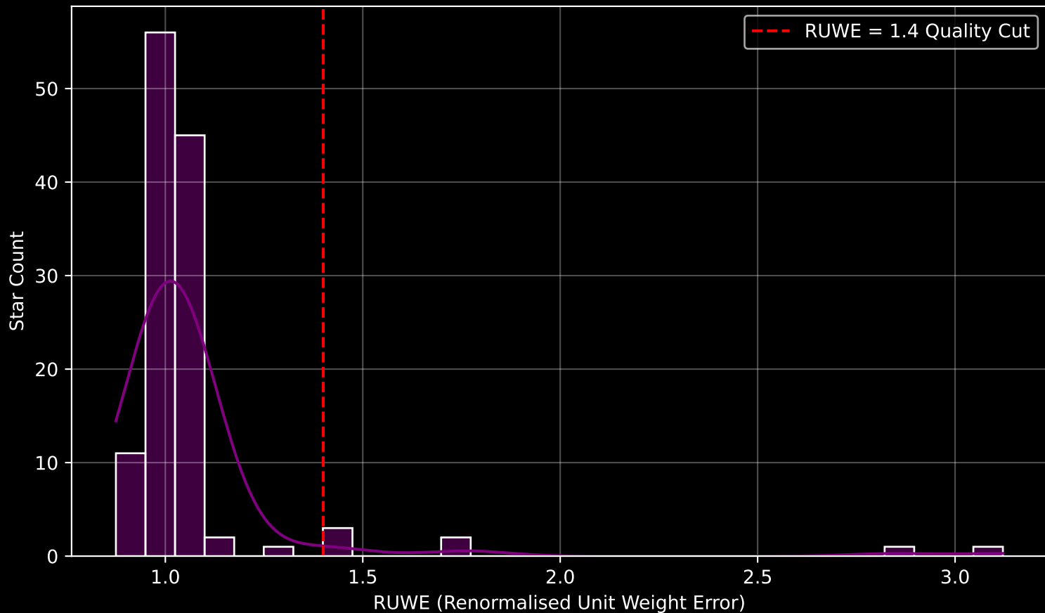
Gaia Cluster: [Muzzio_1] RUWE Distribution (n= 122)
