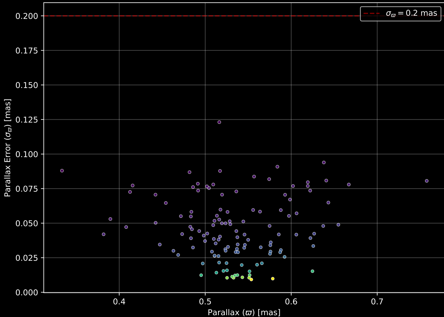
Gaia Cluster: [Muzzio_1] Parallax Quality (n= 124)
