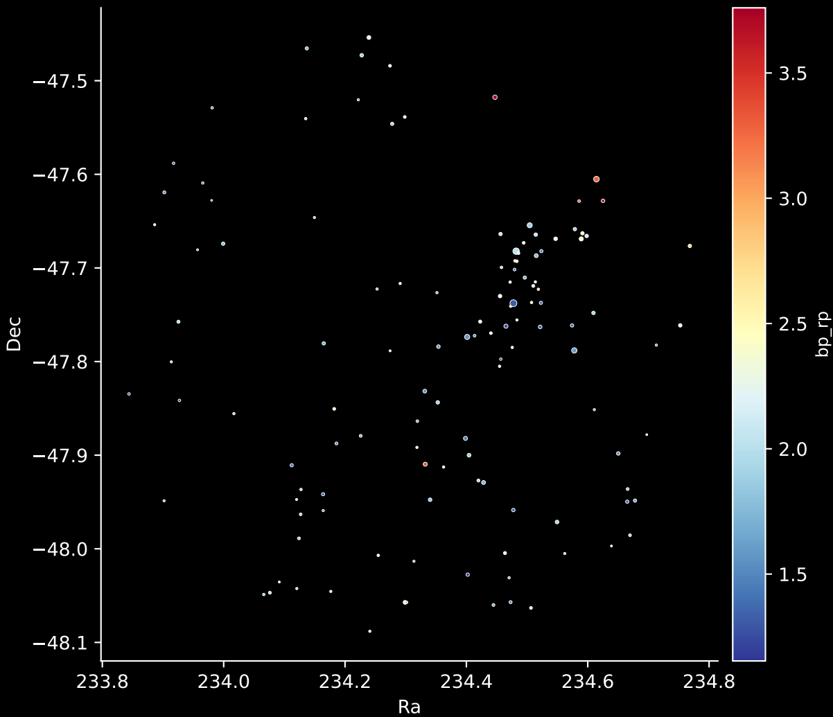
Gaia Cluster: [Muzzio_1] Stars: 124
