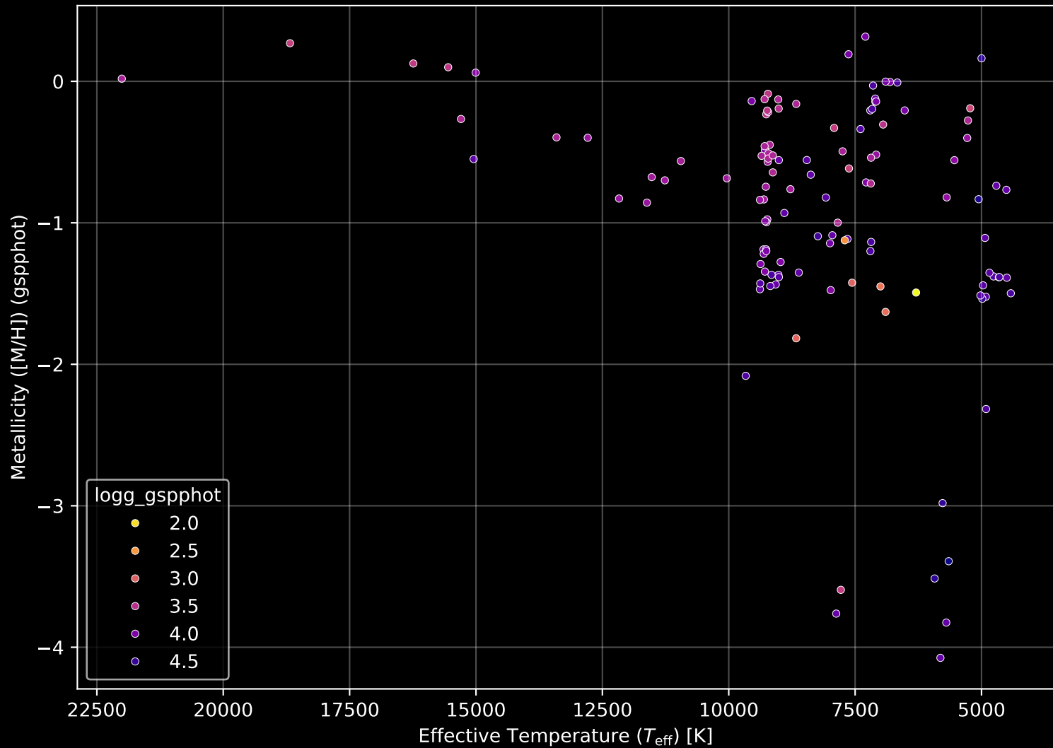
Gaia Cluster: [Muzzio_1] Stellar Population Parameters (n= 124)
