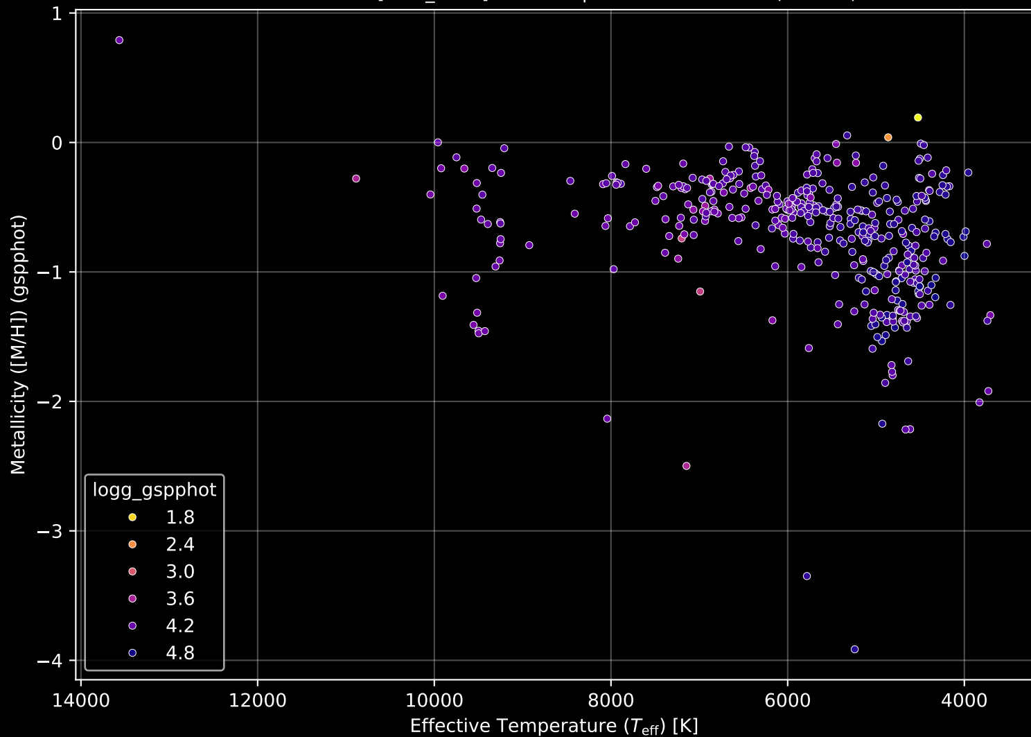
Gaia Cluster: [NGC_1027] Stellar Population Parameters (n= 417)
