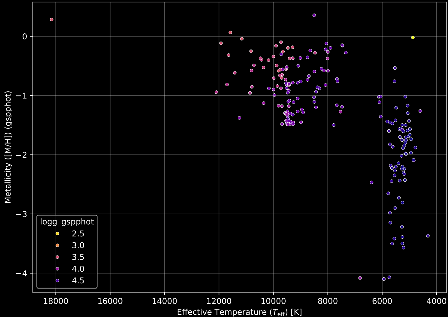
Gaia Cluster: [NGC_103] Stellar Population Parameters (n= 207)
