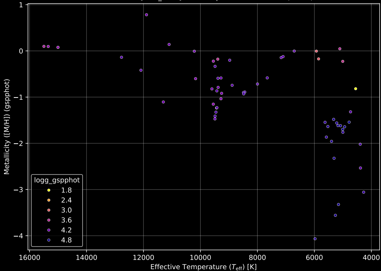
Gaia Cluster: [NGC_1220] Stellar Population Parameters (n= 62)
