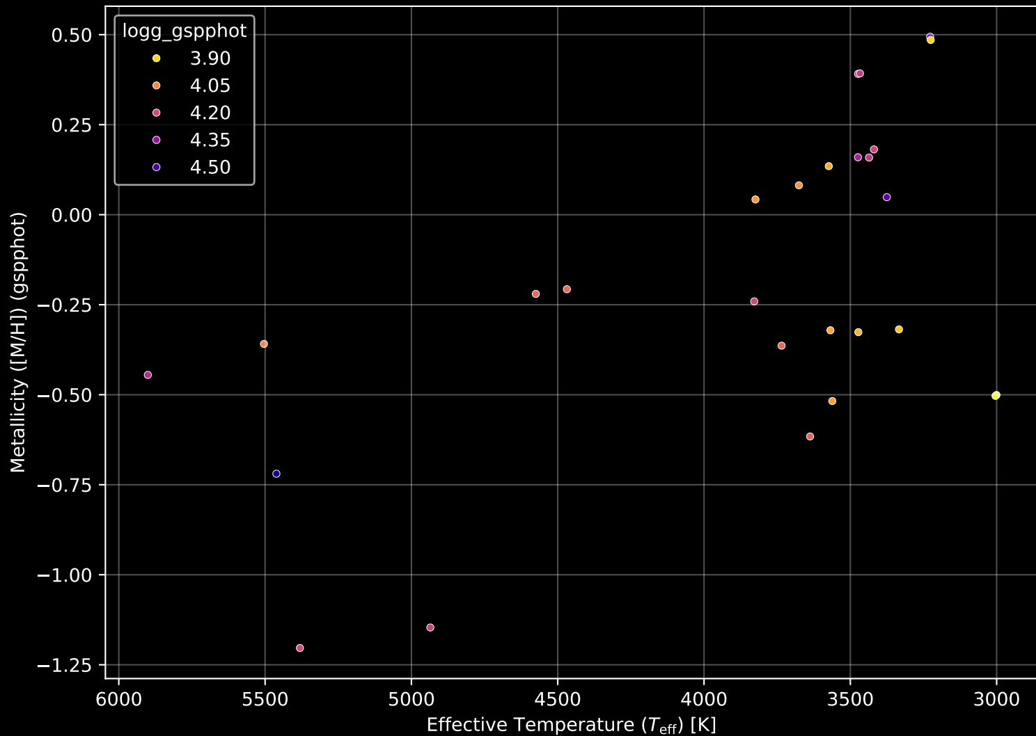
Gaia Cluster: [NGC_1333] Stellar Population Parameters (n= 27)
