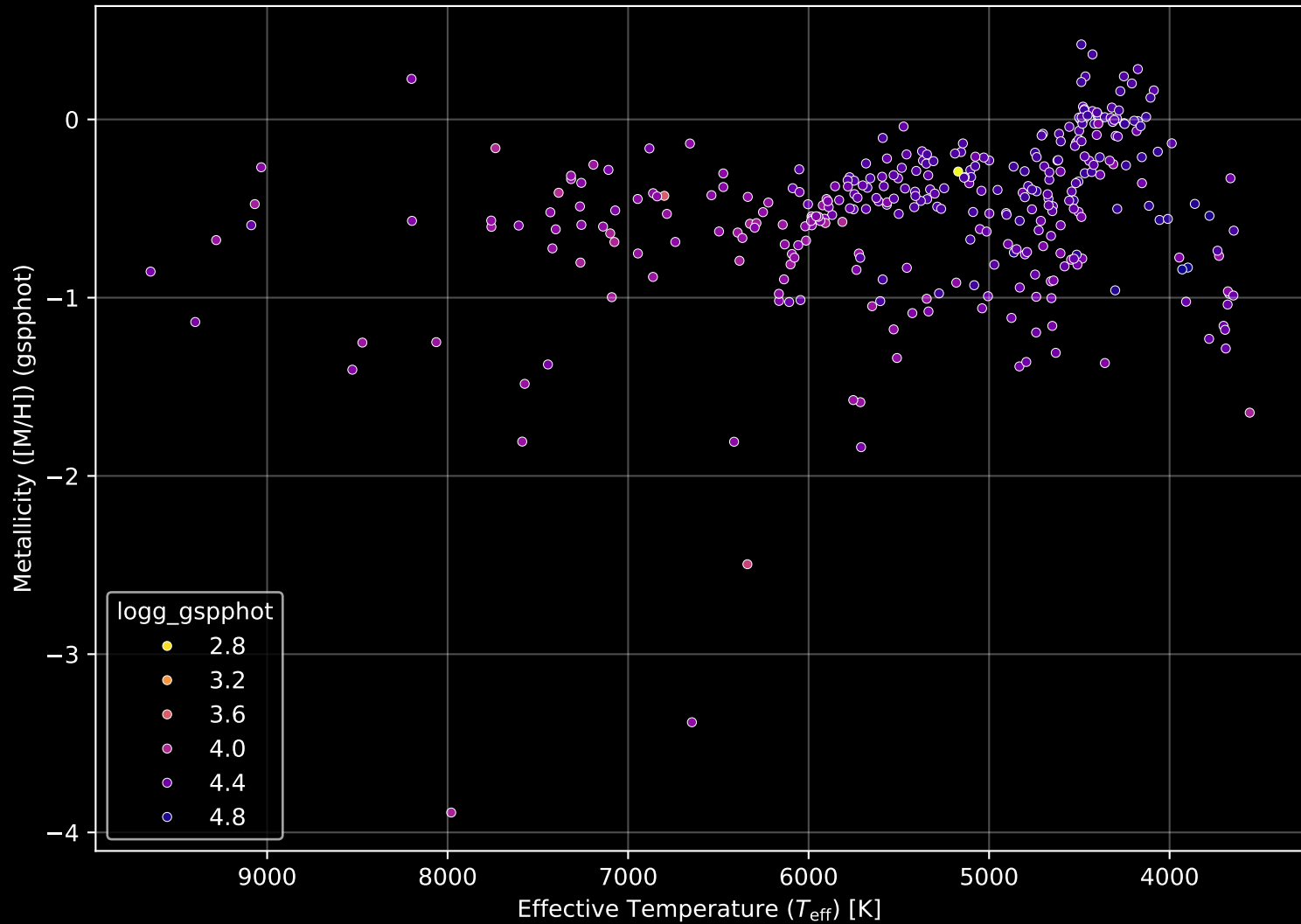
Gaia Cluster: [NGC_1342] Stellar Population Parameters (n= 339)
