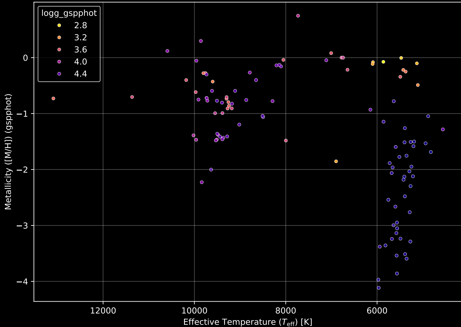
Gaia Cluster: [NGC_136] Stellar Population Parameters (n= 112)
