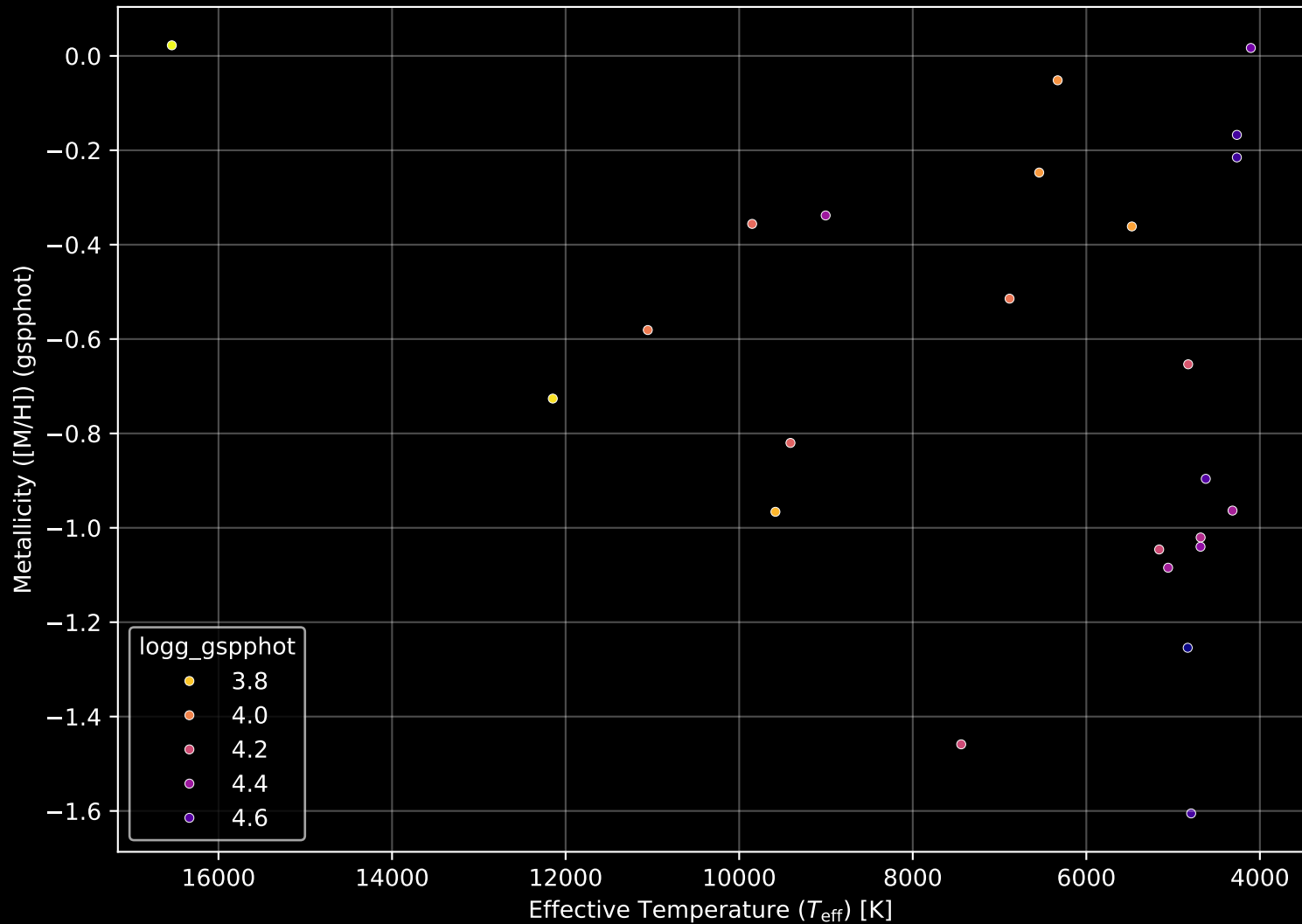
Gaia Cluster: [NGC 1444] Stellar Population Parameters (n= 24)
