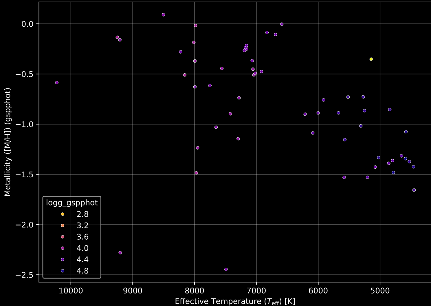
Gaia Cluster: [NGC_1496] Stellar Population Parameters (n= 57)
