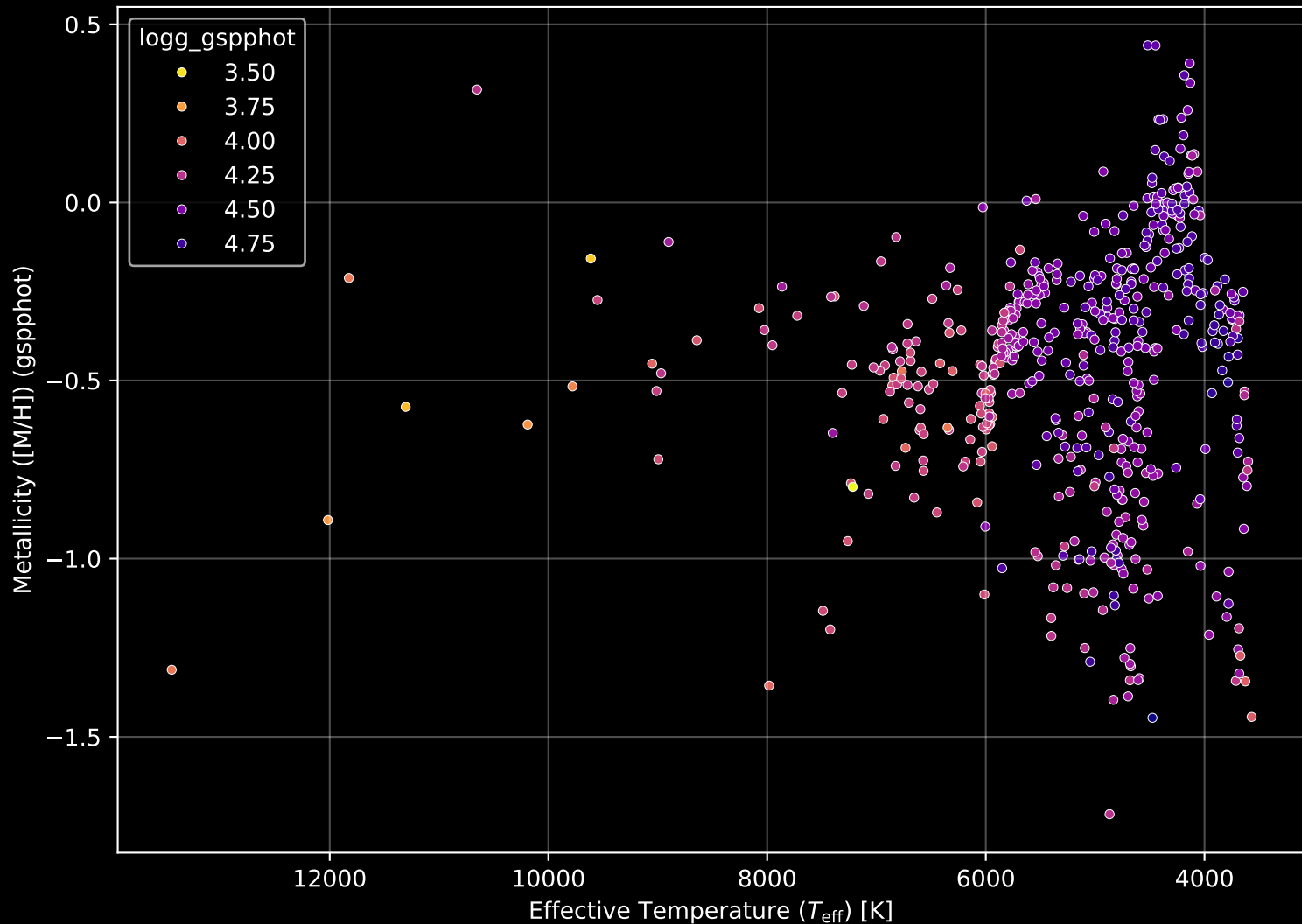
Gaia Cluster: [NGC_1647] Stellar Population Parameters (n= 547)
