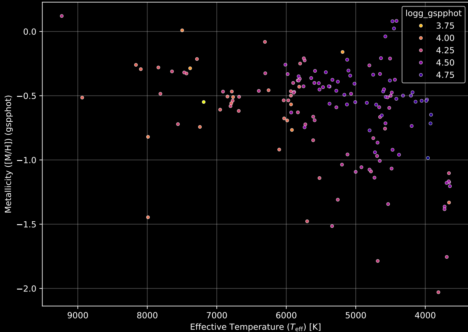
Gaia Cluster: [NGC_1758] Stellar Population Parameters (n= 153)
