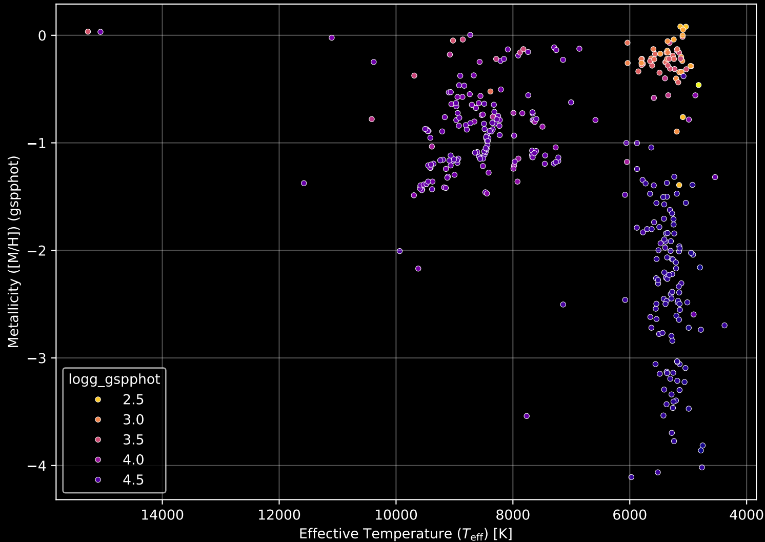
Gaia Cluster: [NGC_1798] Stellar Population Parameters (n= 349)
