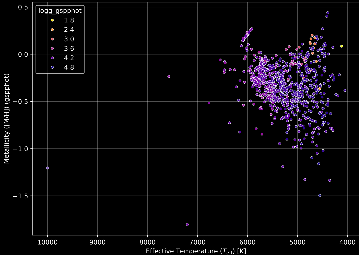
Gaia Cluster: [NGC_188] Stellar Population Parameters (n= 804)
