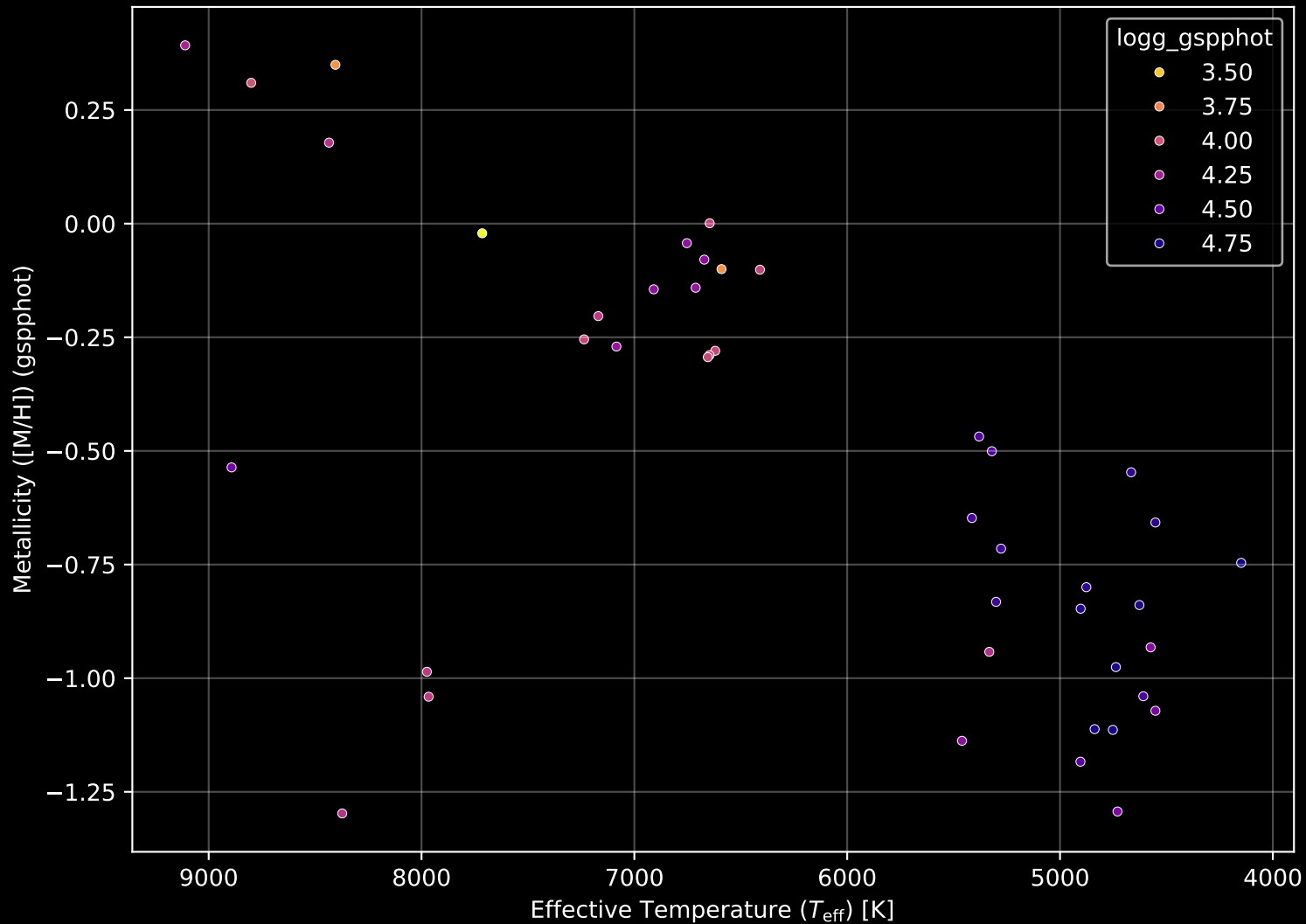
Gaia Cluster: [NGC_189] Stellar Population Parameters (n= 43)
