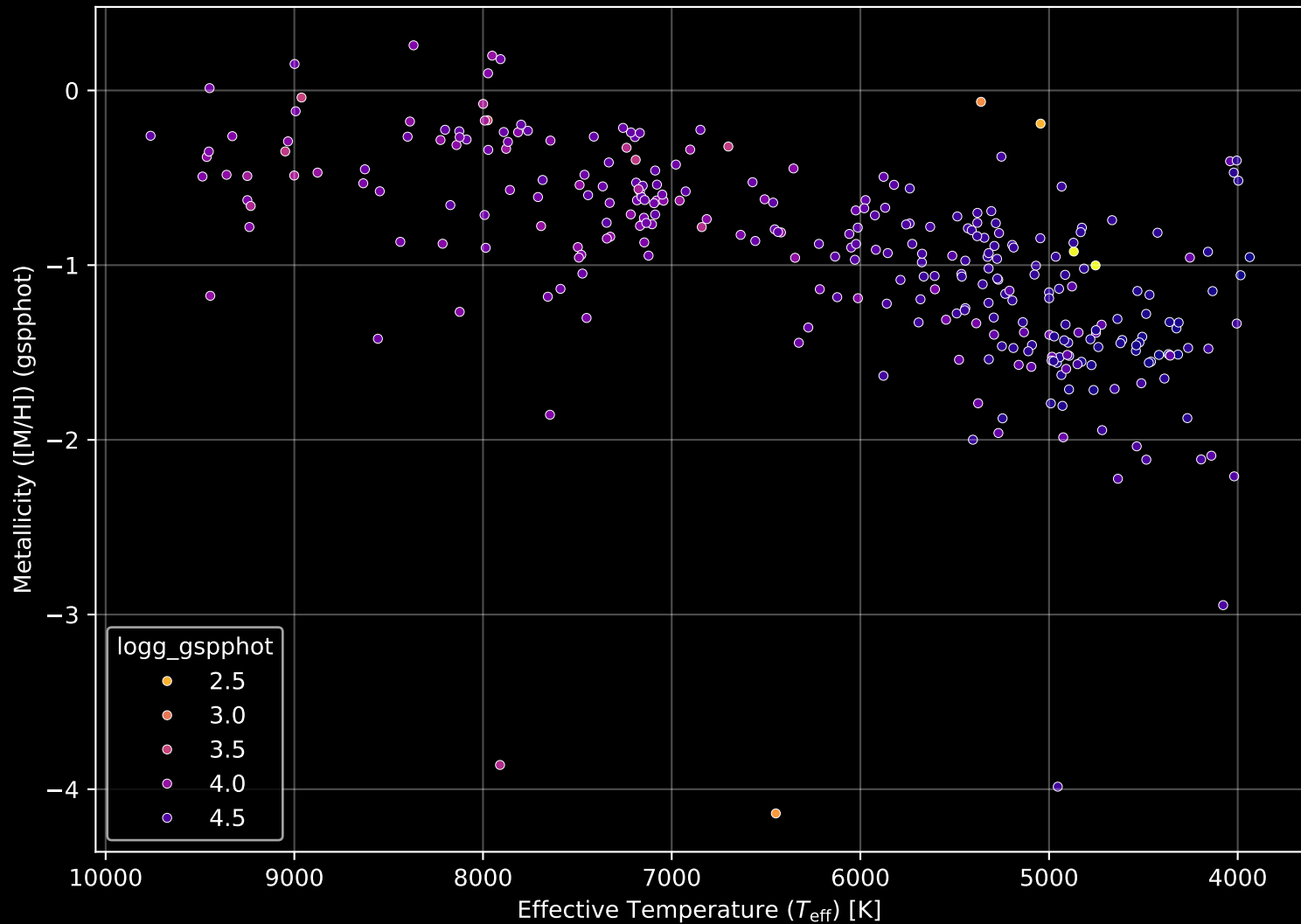
Gaia Cluster: [NGC_1907] Stellar Population Parameters (n= 301)
