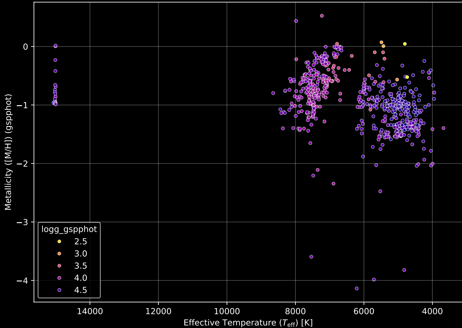
Gaia Cluster: [NGC_2112] Stellar Population Parameters (n= 672)
