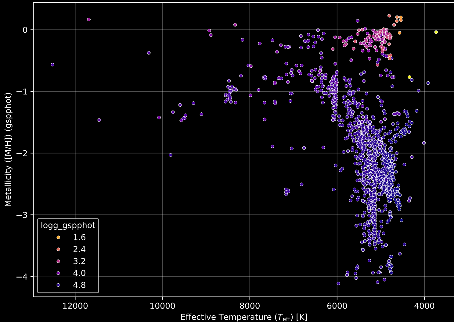
Gaia Cluster: [NGC_2141] Stellar Population Parameters (n= 1357)
