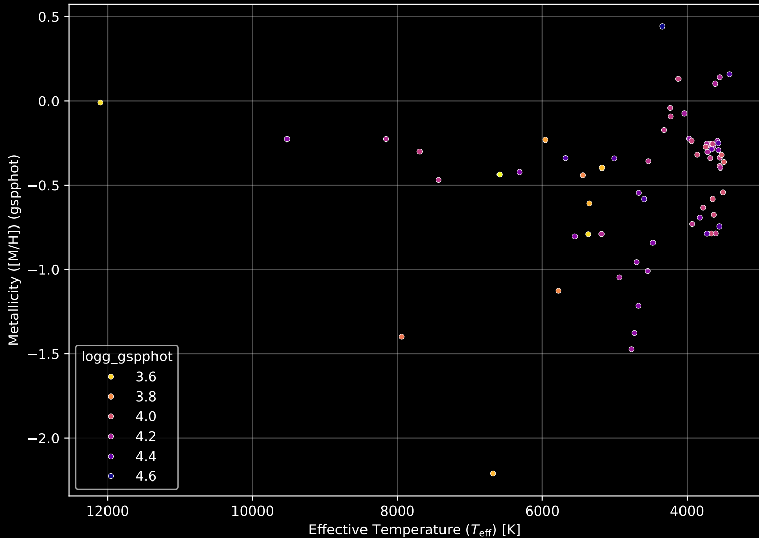
Gaia Cluster: [NGC_2183] Stellar Population Parameters (n= 68)
