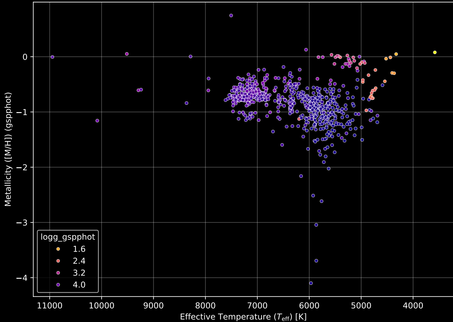
Gaia Cluster: [NGC_2204] Stellar Population Parameters (n= 717)
