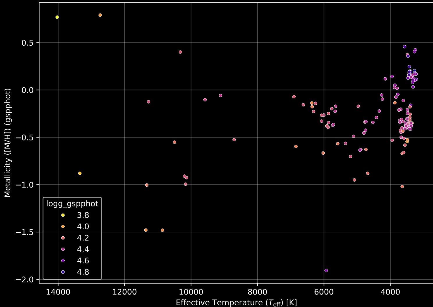
Gaia Cluster: [NGC_2232] Stellar Population Parameters (n= 171)
