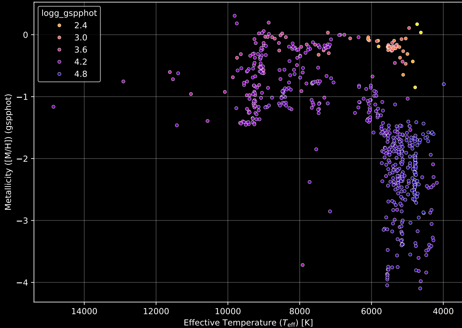
Gaia Cluster: [NGC_2236] Stellar Population Parameters (n= 601)
