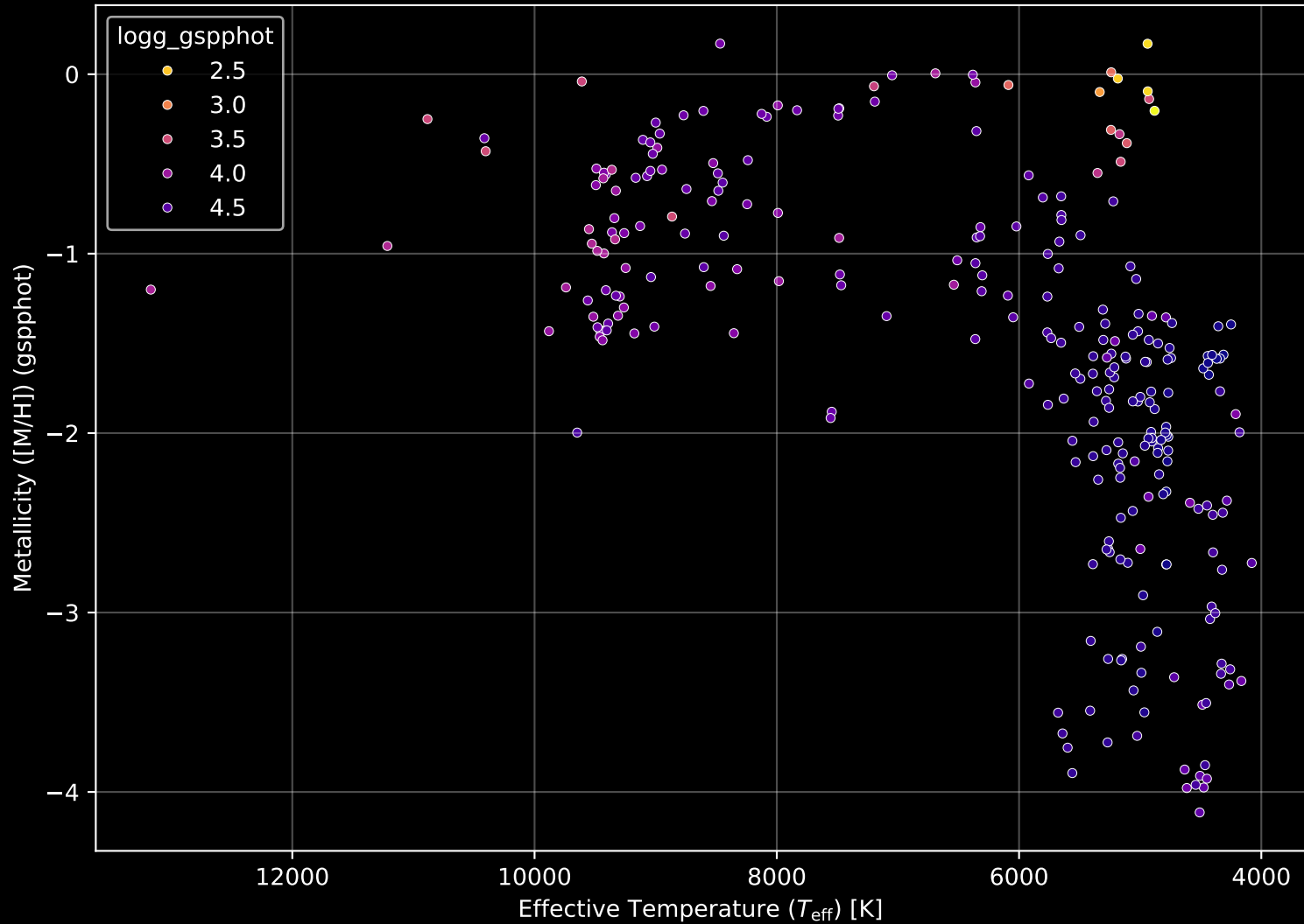
Gaia Cluster: [NGC_2254] Stellar Population Parameters (n= 277)
