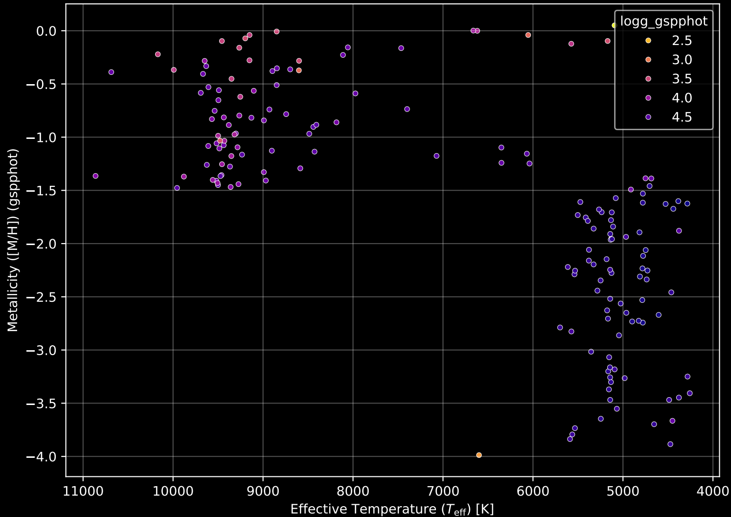
Gaia Cluster: [NGC_2259] Stellar Population Parameters (n= 167)
