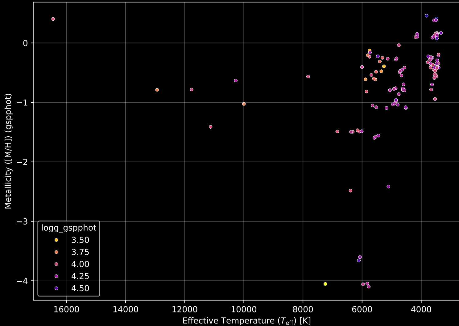
Gaia Cluster: [NGC_2264] Stellar Population Parameters (n= 124)
