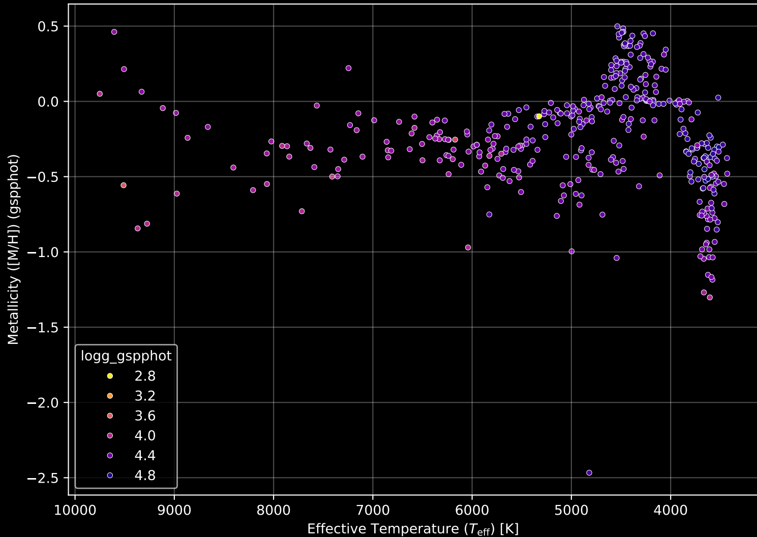
Gaia Cluster: [NGC_2281] Stellar Population Parameters (n= 395)
