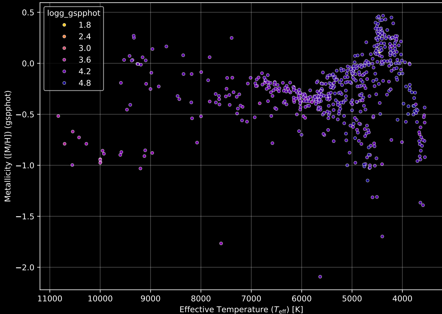
Gaia Cluster: [NGC_2287] Stellar Population Parameters (n= 574)
