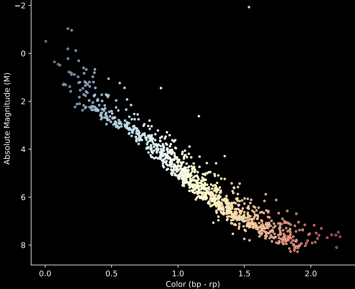
Gaia Cluster: [NGC_2323] Stars (n= 1160) Hertzprung-Russel Diagram
