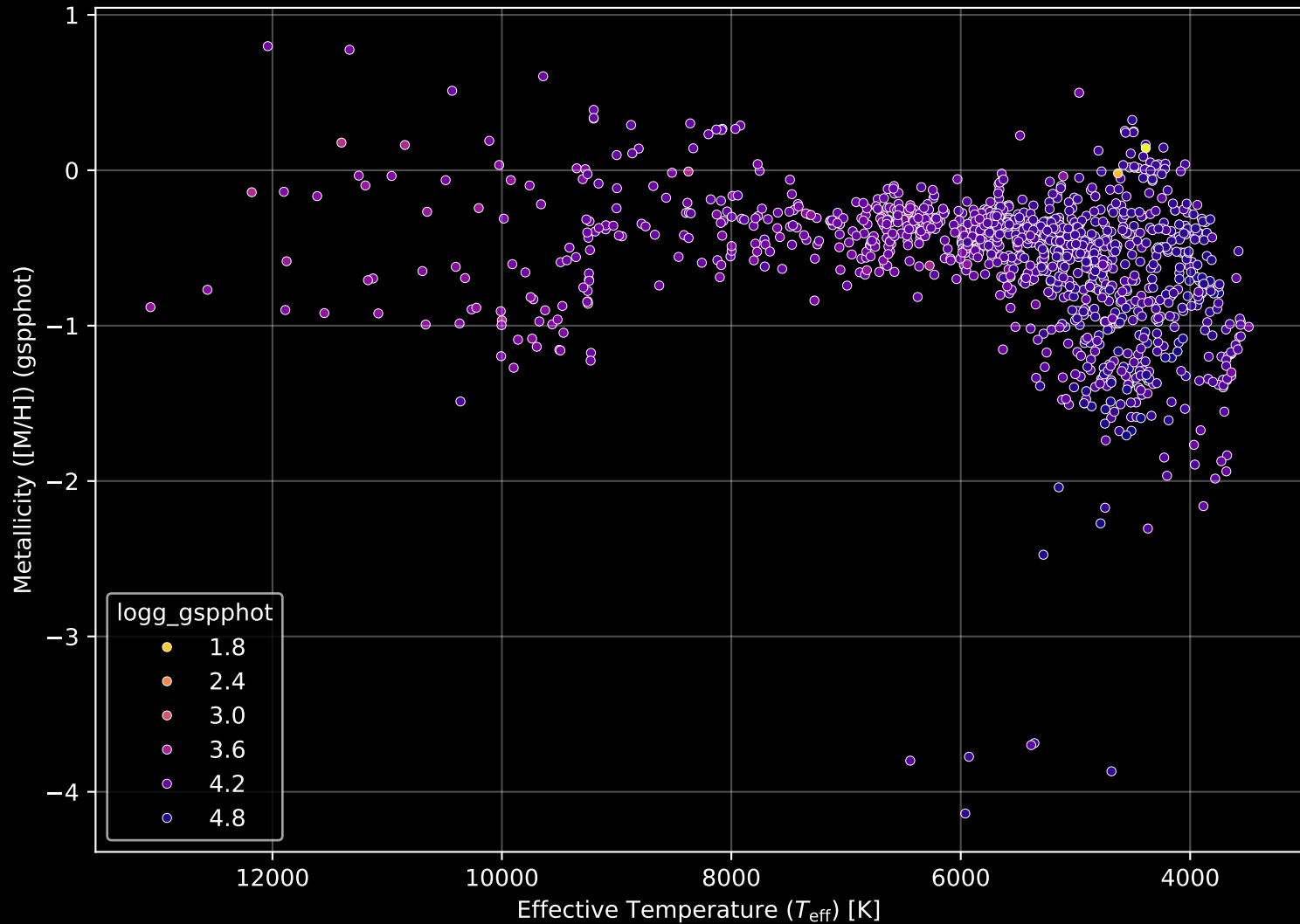
Gaia Cluster: [NGC_2323] Stellar Population Parameters (n= 1160)
