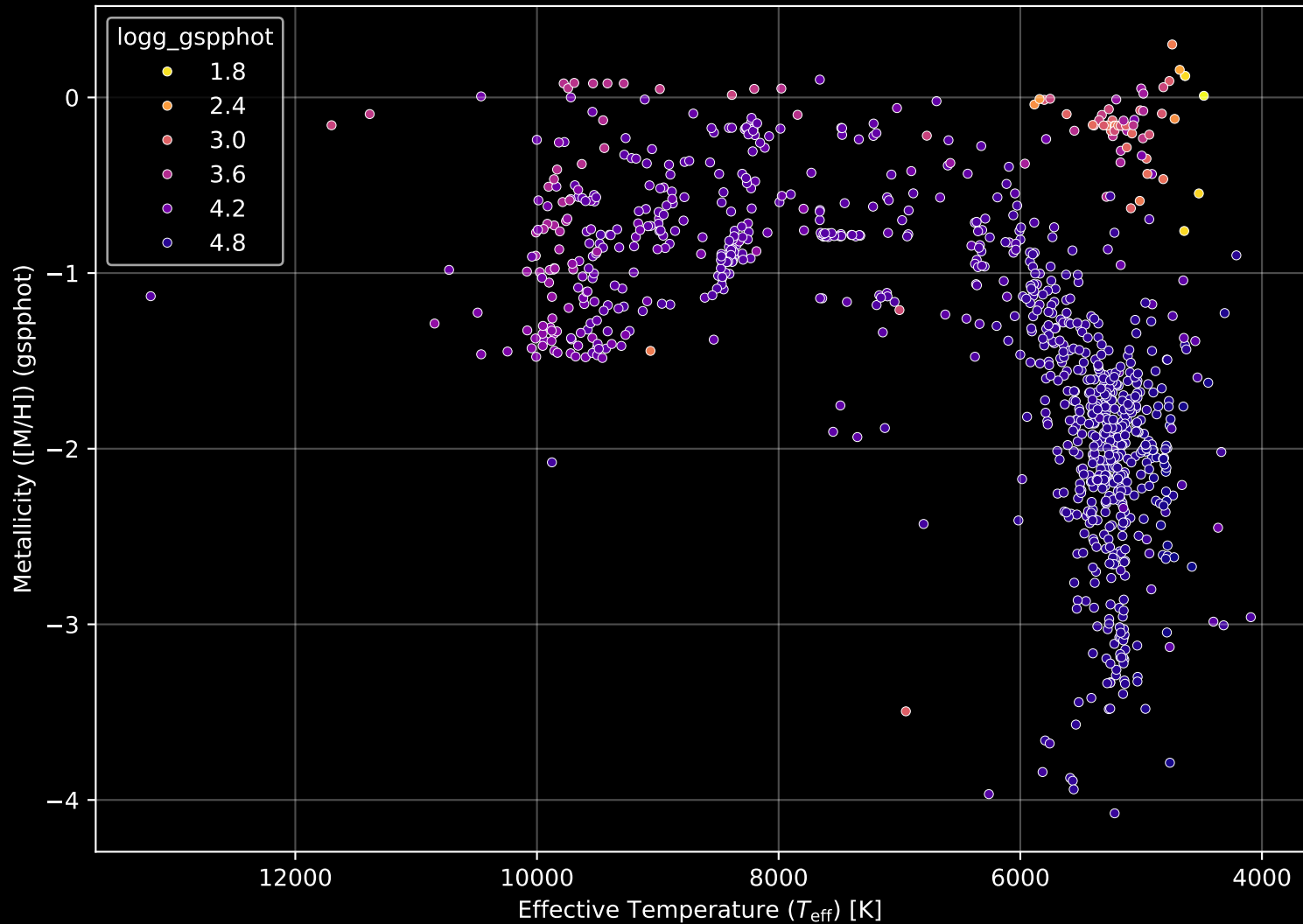
Gaia Cluster: [NGC_2324] Stellar Population Parameters (n= 995)
