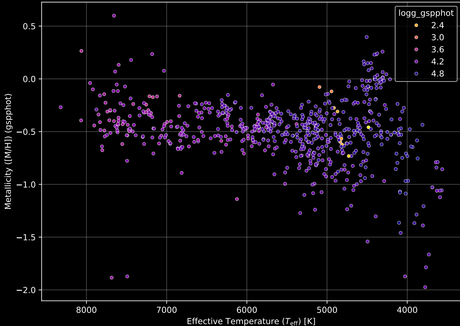
Gaia Cluster: [NGC_2360] Stellar Population Parameters (n= 650)
