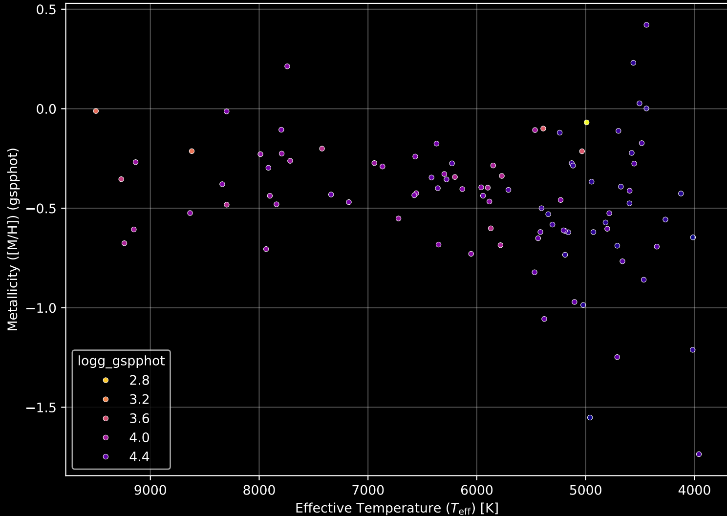
Gaia Cluster: [NGC_2374] Stellar Population Parameters (n= 95)
