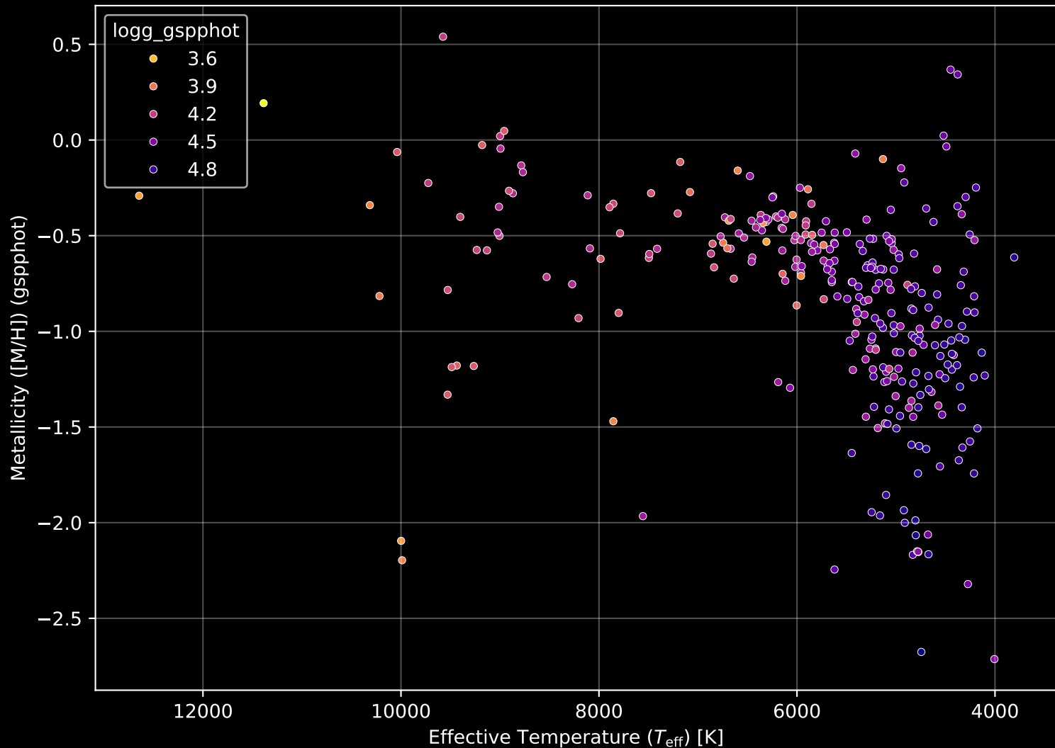
Gaia Cluster: [NGC_2396] Stellar Population Parameters (n= 301)
