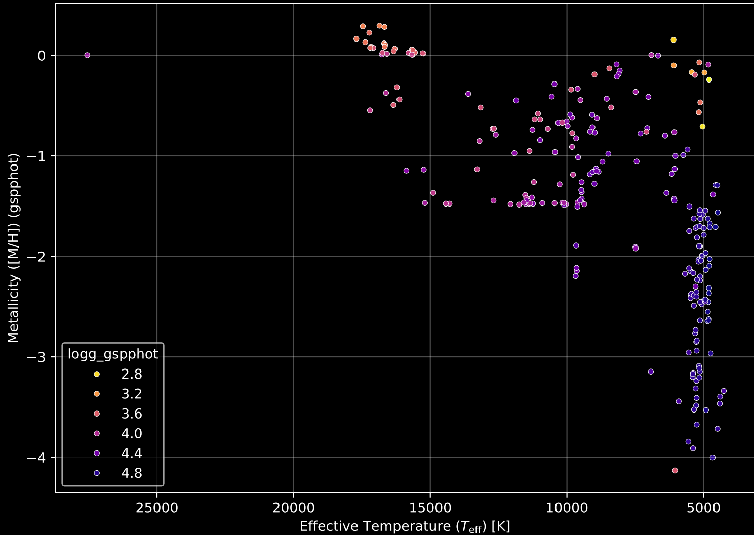
Gaia Cluster: [NGC_2414] Stellar Population Parameters (n= 248)
