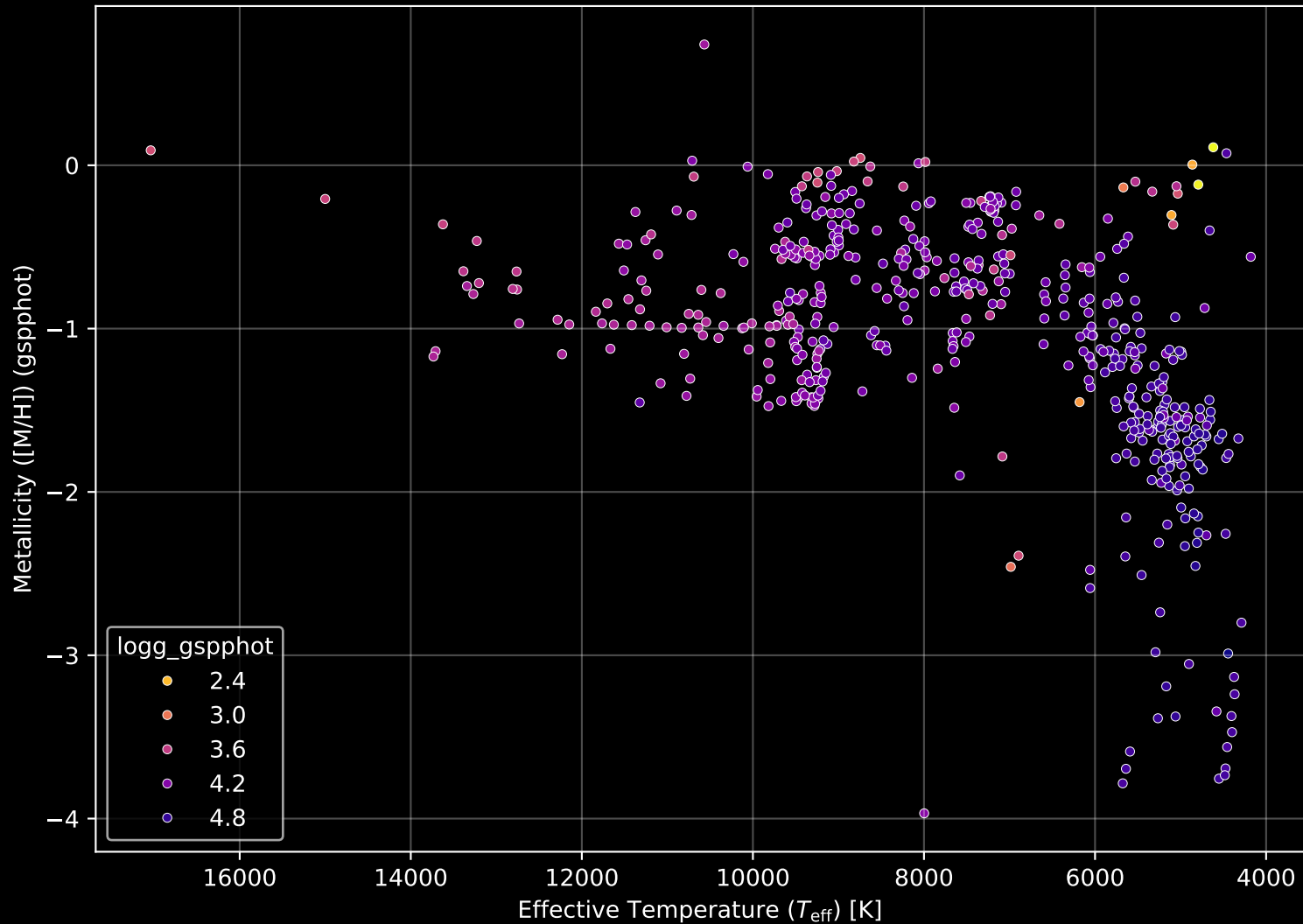
Gaia Cluster: [NGC_2421] Stellar Population Parameters (n= 544)
