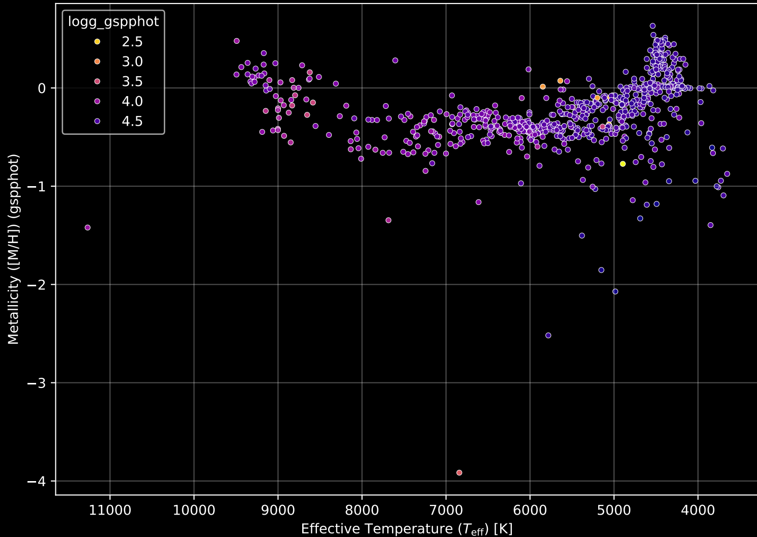
Gaia Cluster: [NGC_2447] Stellar Population Parameters (n= 730)
