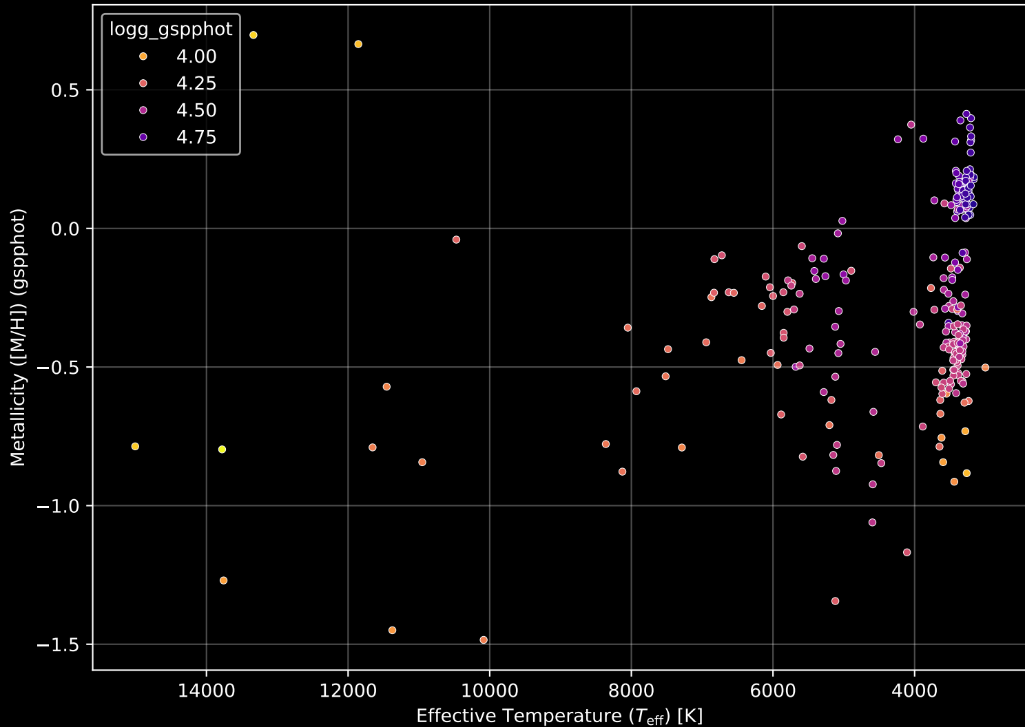
Gaia Cluster: [NGC_2451A] Stellar Population Parameters (n= 289)
