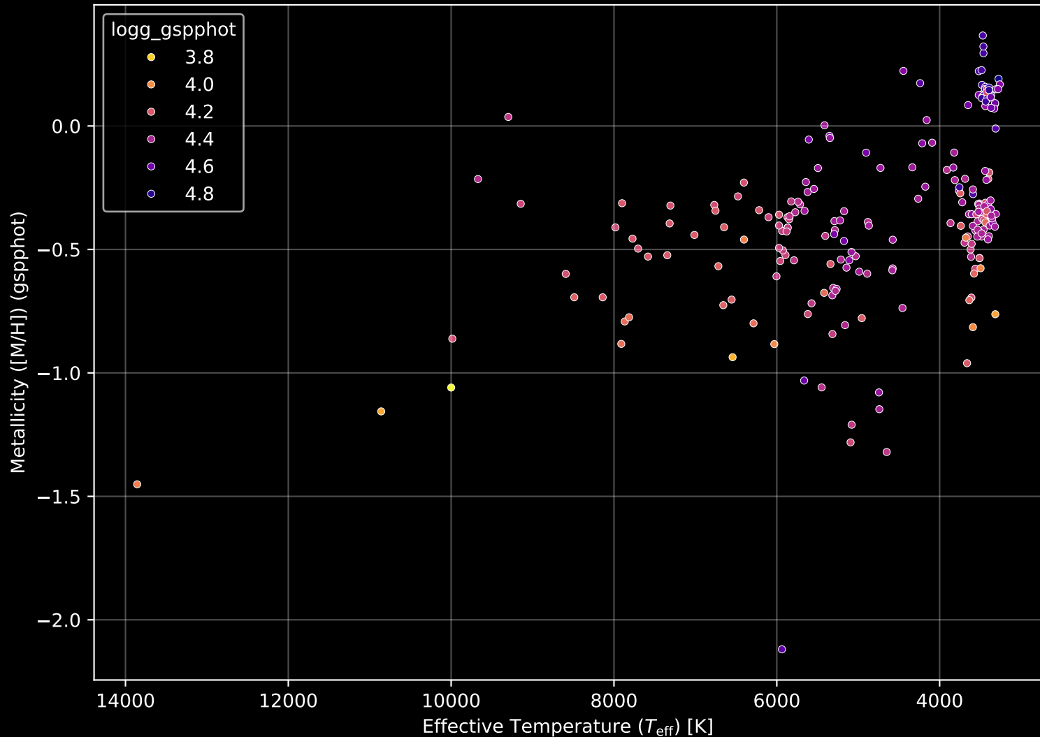
Gaia Cluster: [NGC_2451B] Stellar Population Parameters (n= 236)
