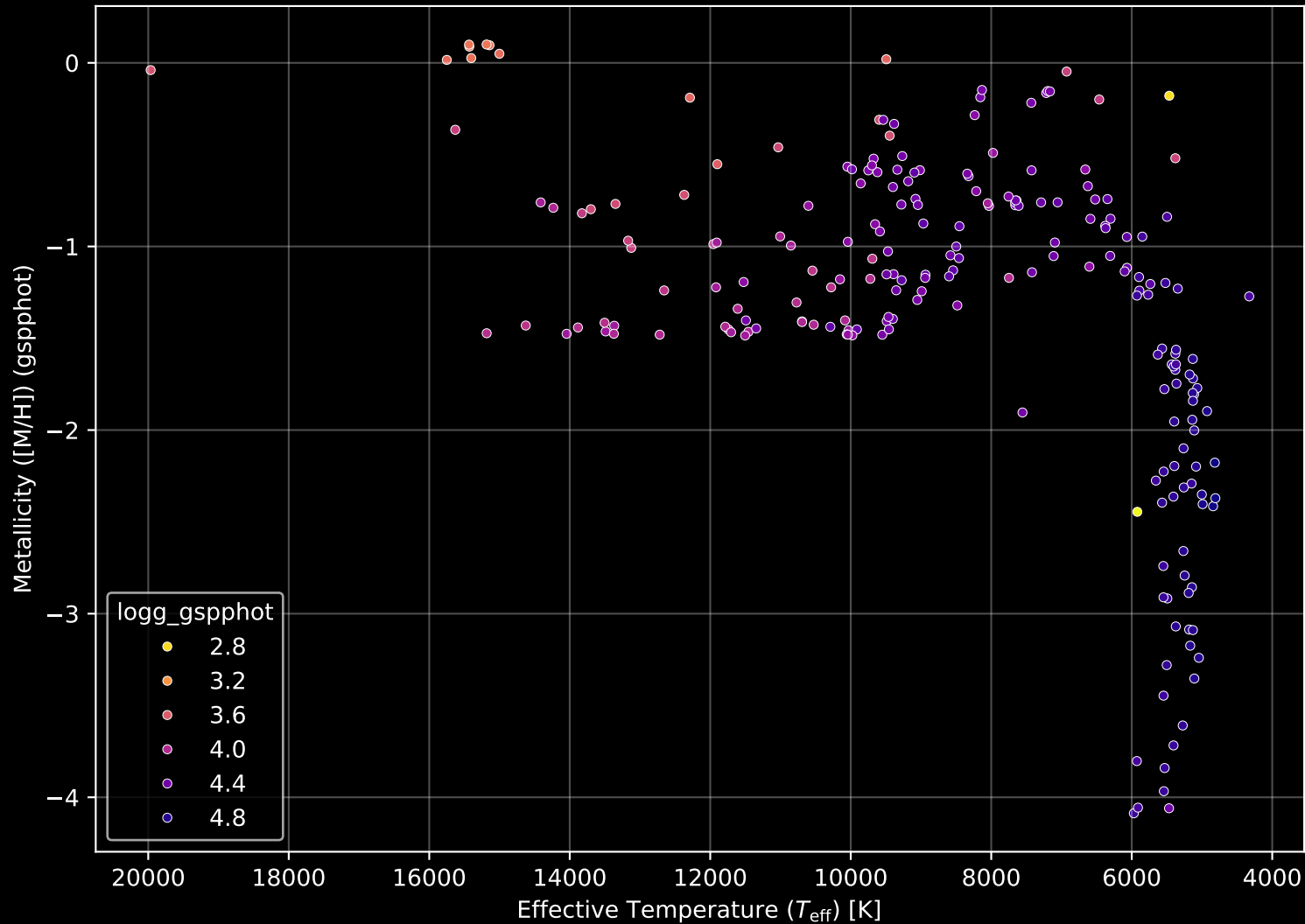
Gaia Cluster: [NGC_2453] Stellar Population Parameters (n= 220)
