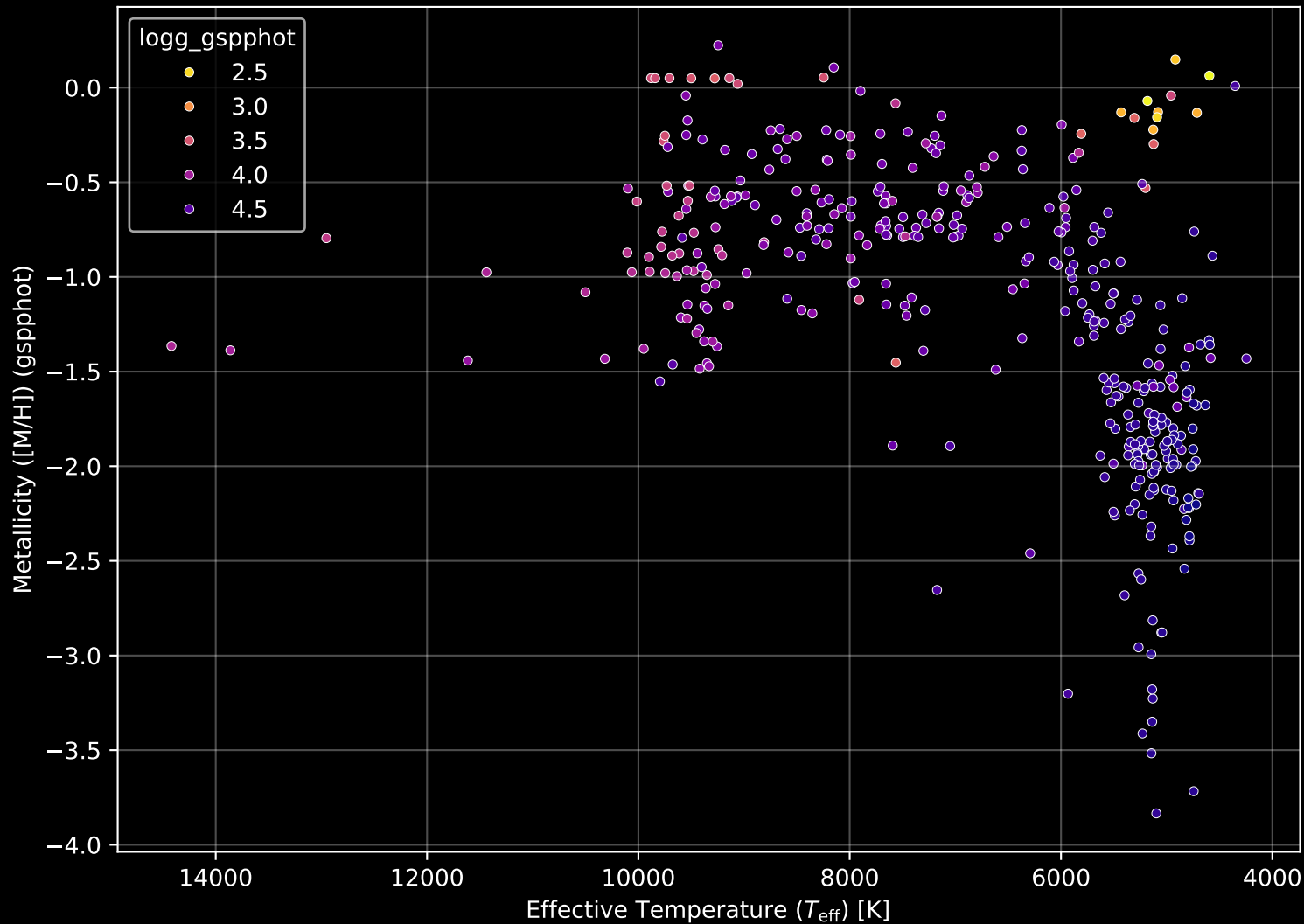
Gaia Cluster: [NGC_2455] Stellar Population Parameters (n= 412)
