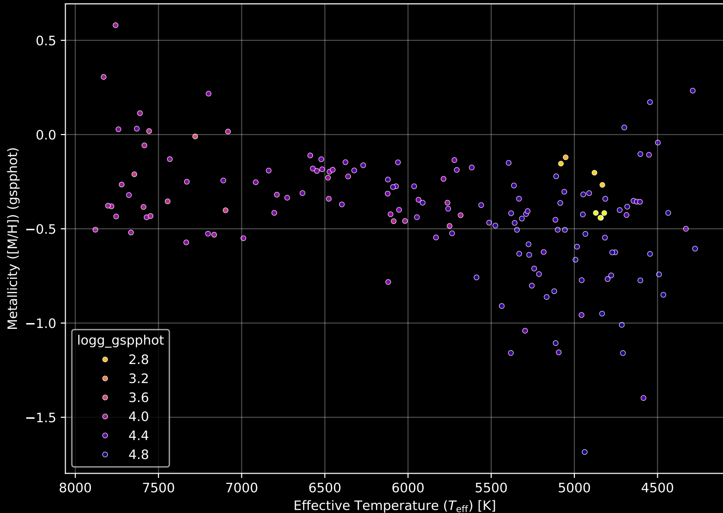
Gaia Cluster: [NGC_2479] Stellar Population Parameters (n= 153)
