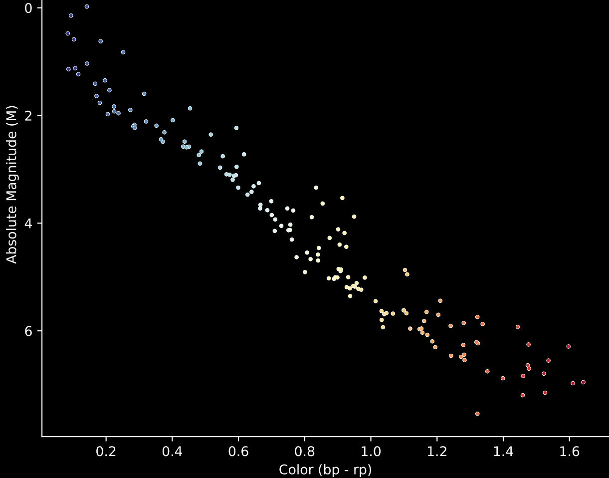
Hertzprung-Russel Diagram
