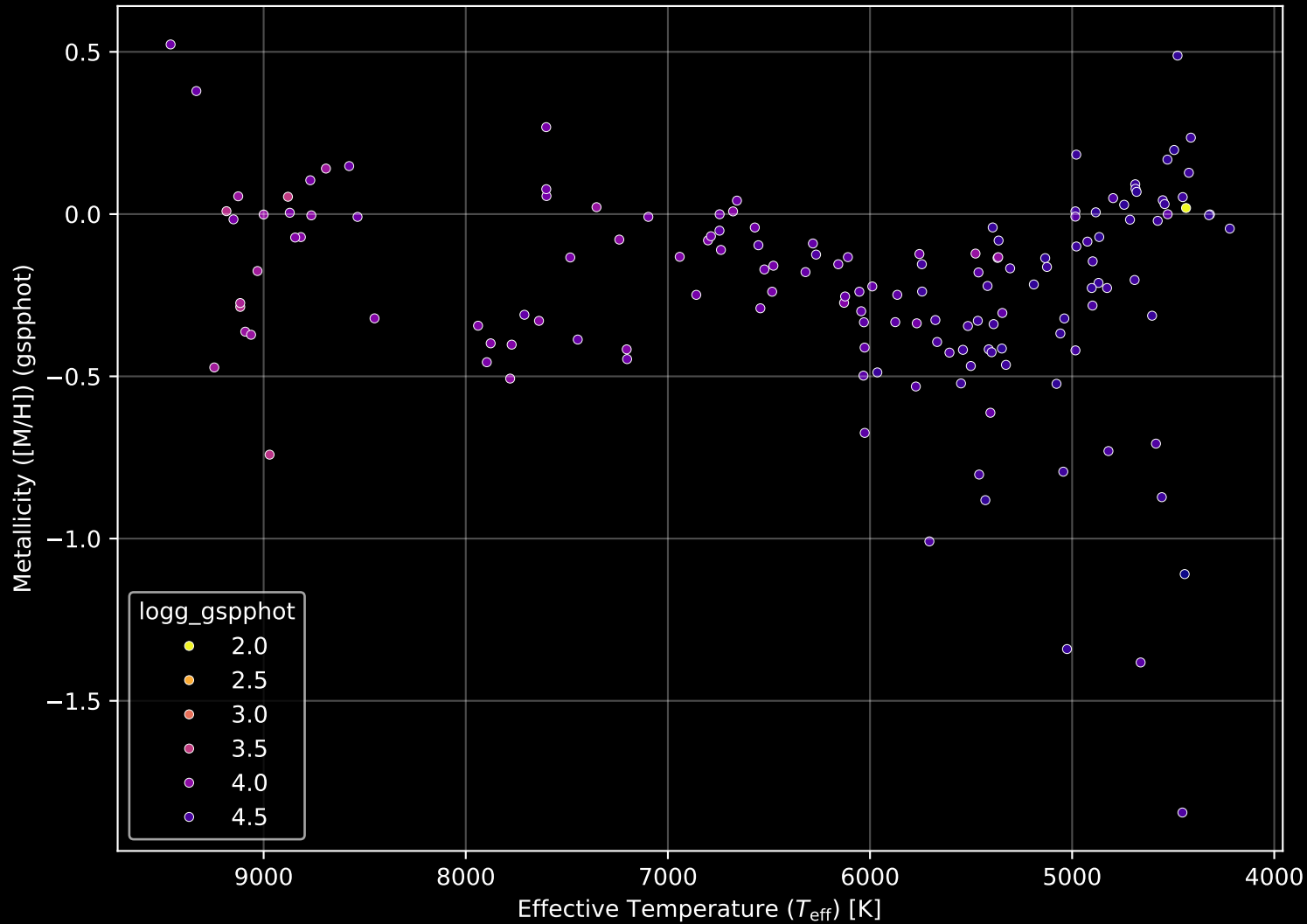
Gaia Cluster: [NGC_2482] Stellar Population Parameters (n= 152)
