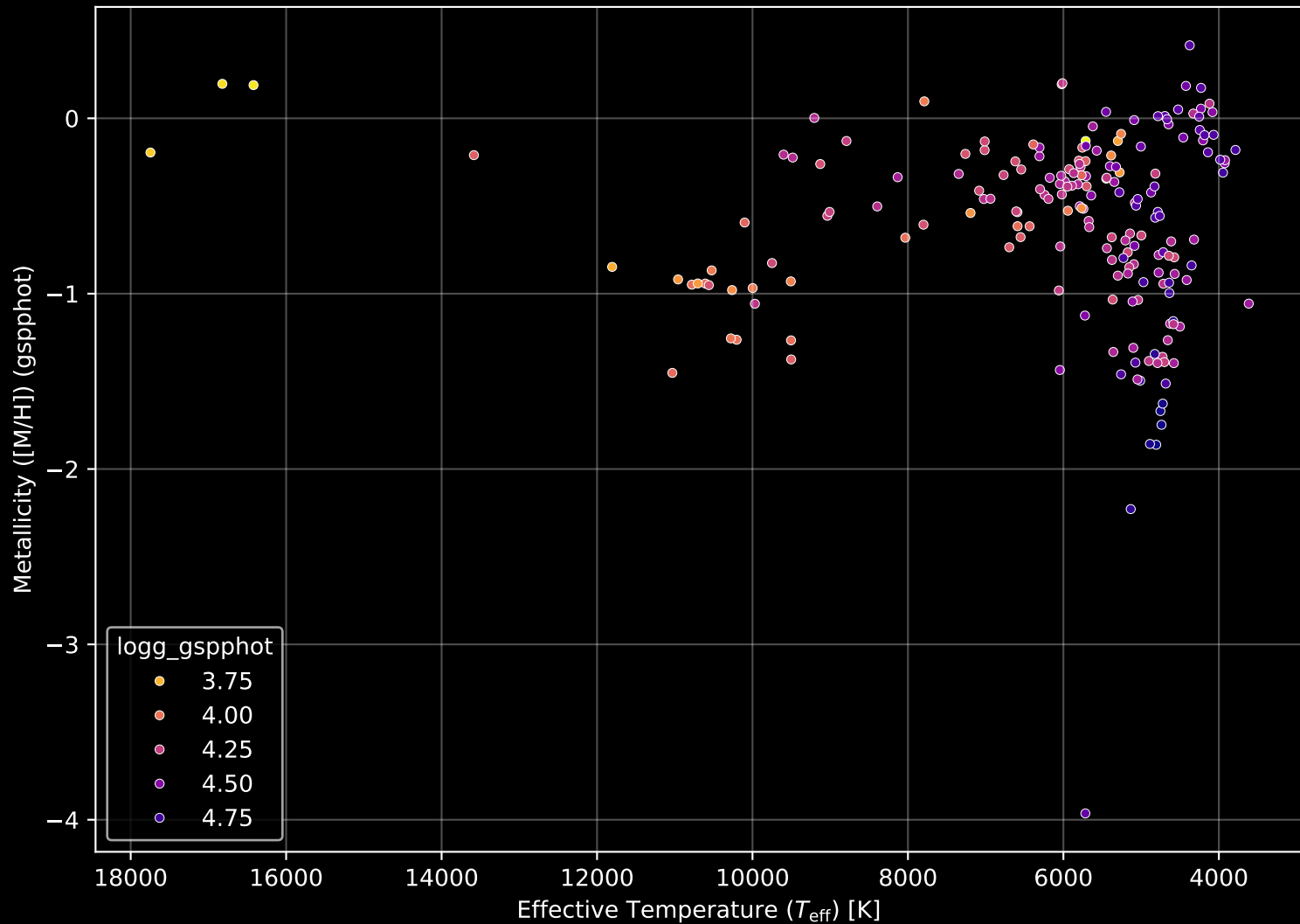
Gaia Cluster: [NGC_2571] Stellar Population Parameters (n= 194)
