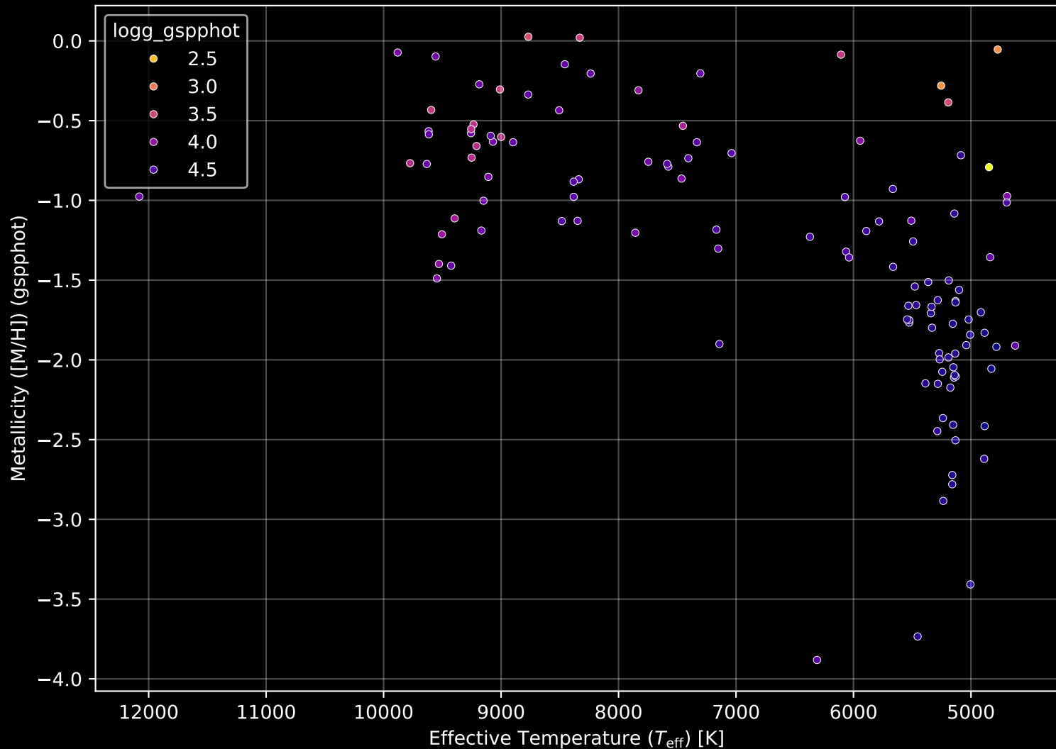
Gaia Cluster: [NGC_2588] Stellar Population Parameters (n= 121)
