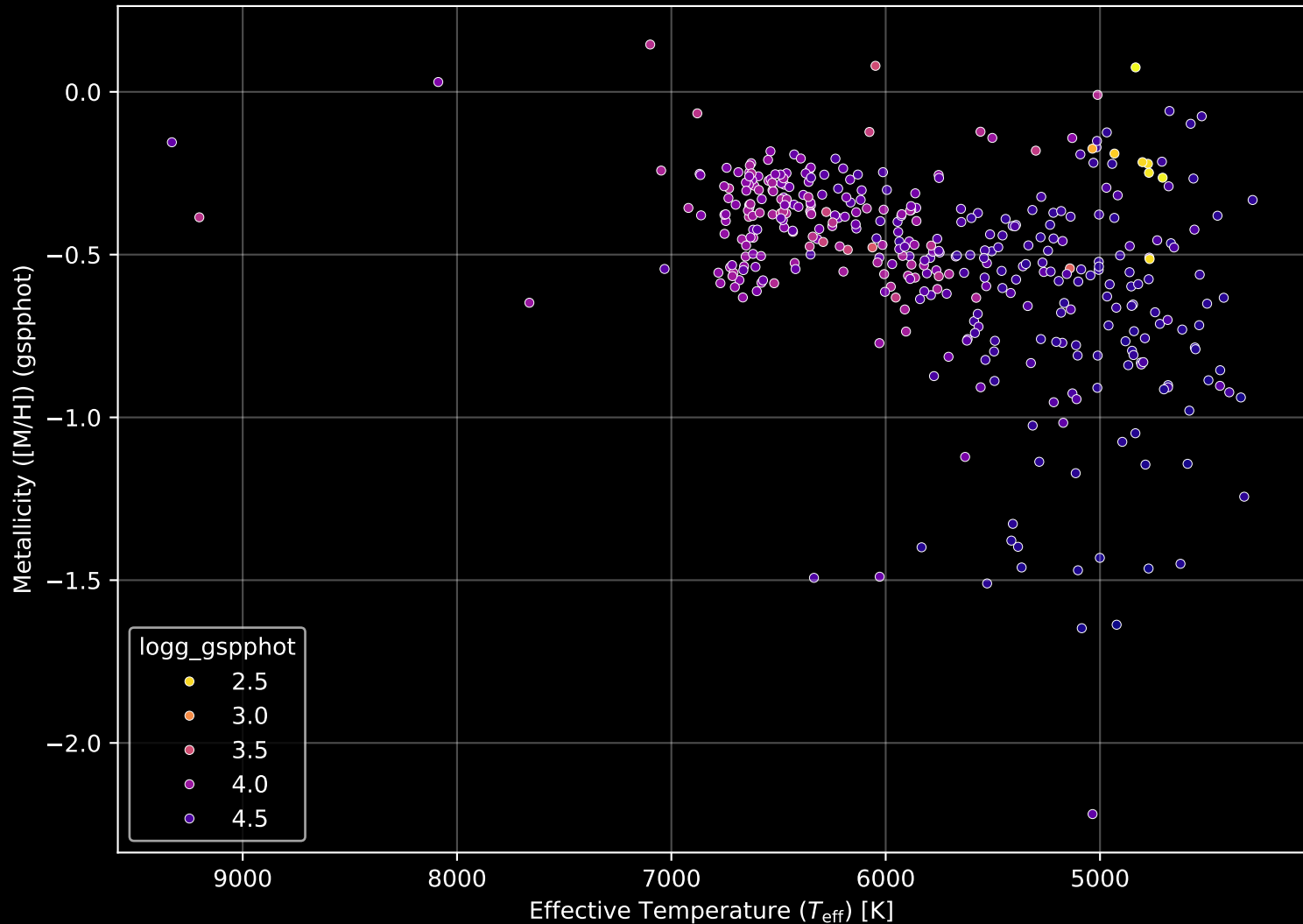
Gaia Cluster: [NGC_2627] Stellar Population Parameters (n= 384)
