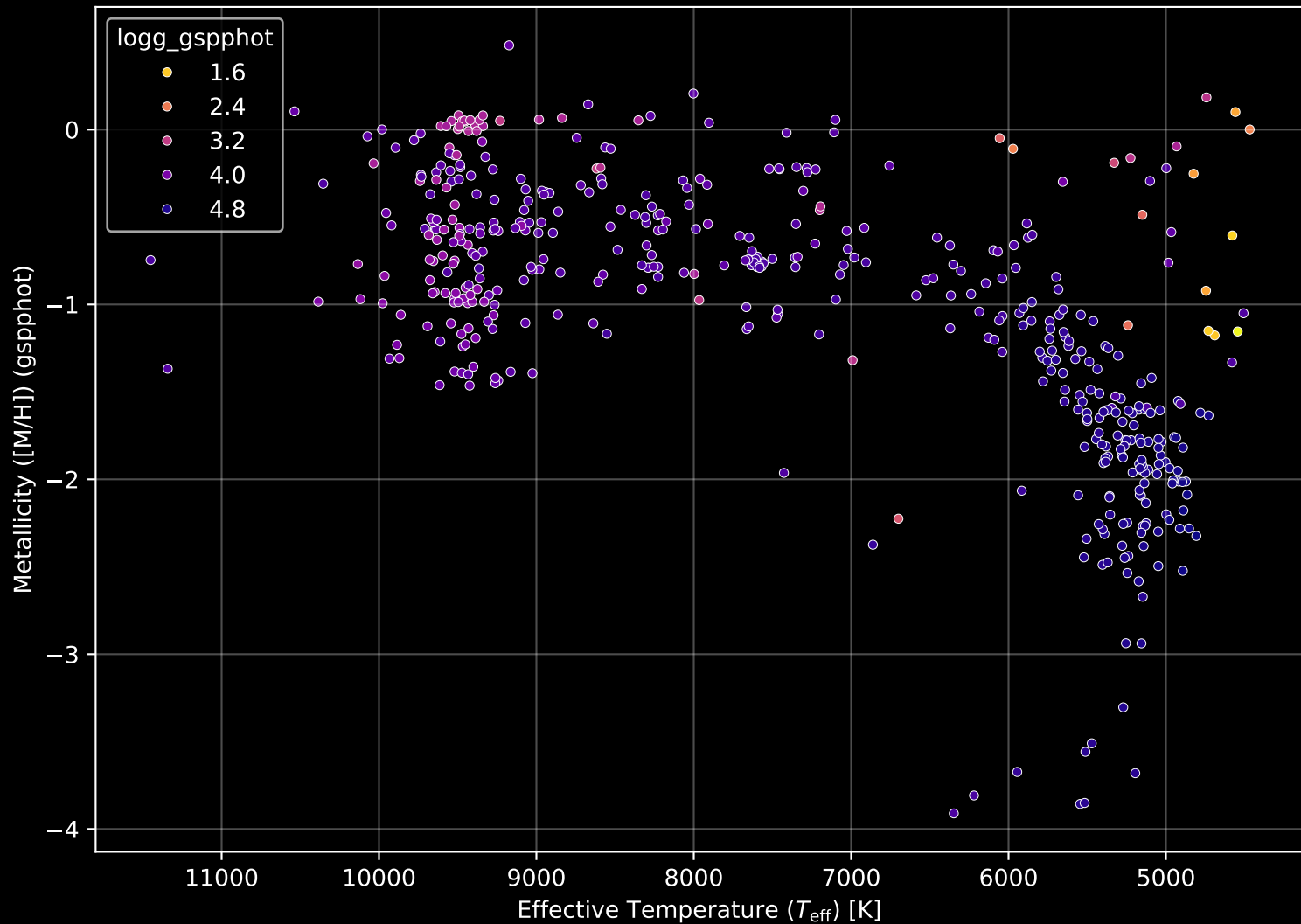
Gaia Cluster: [NGC_2658] Stellar Population Parameters (n= 484)
