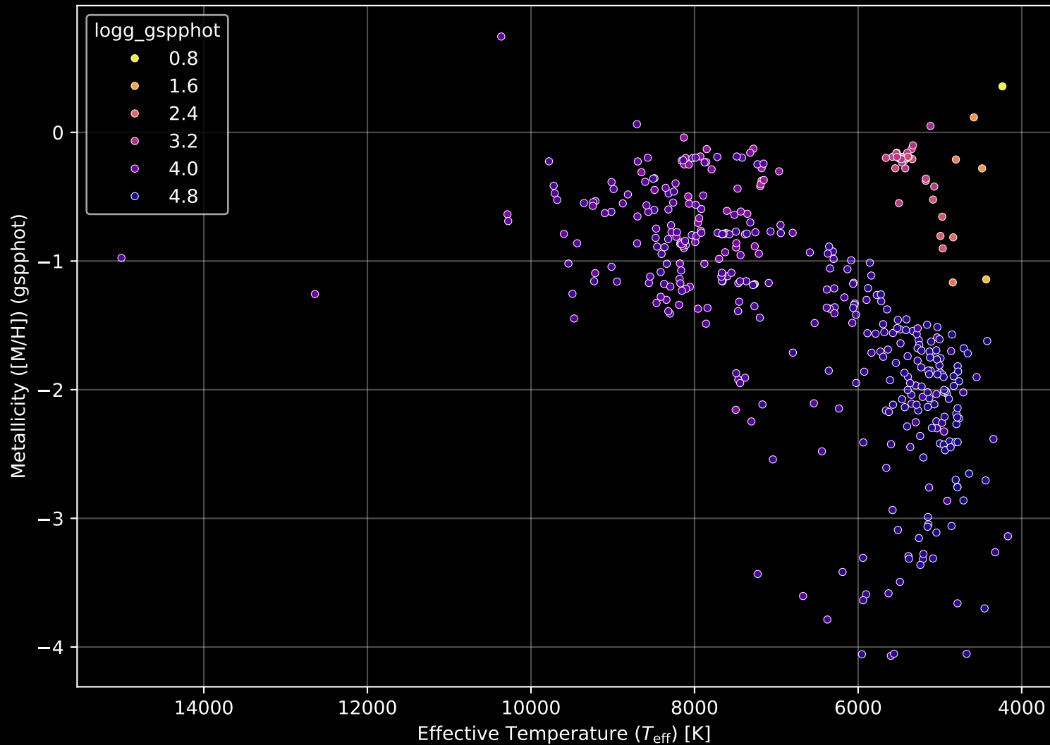
Gaia Cluster: [NGC_2660] Stellar Population Parameters (n= 411)
